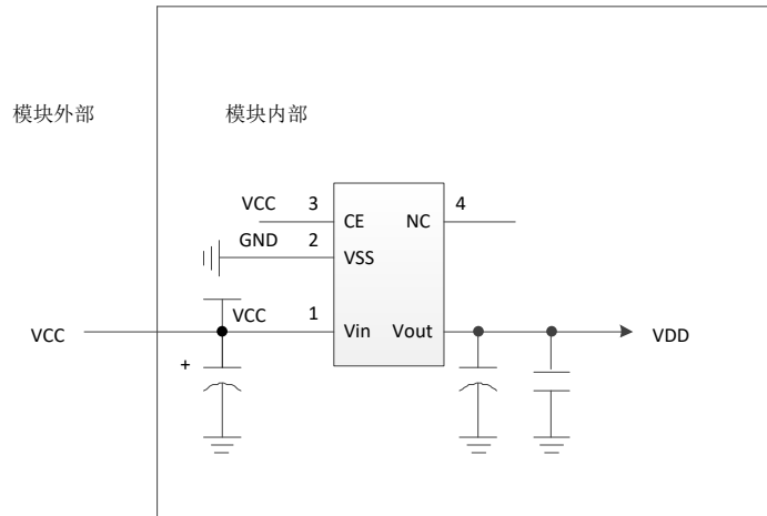
图 5-6 电源 LDO
