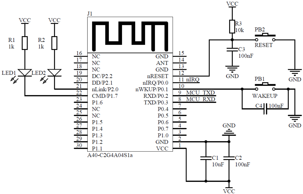
图 5-1 A40-C2G4A04S1a 应用电路
