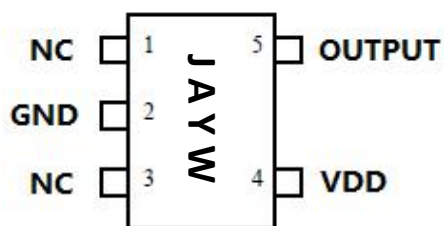
SOT-553 管脚图
