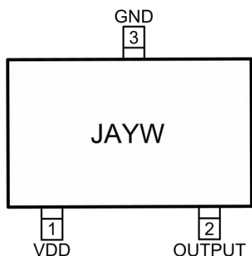
SOT-23 管脚图
