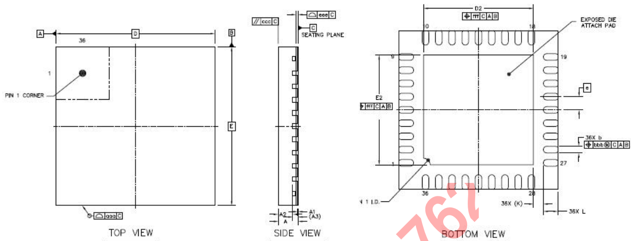
图 27 QFN36 封装
