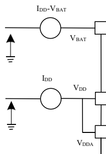
图 11 电流消耗测量方案
