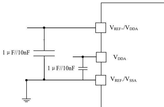
图 25 供电电源和参考电源去藕线路( V_{REF+} 未与 V_{DDA} 相连)
