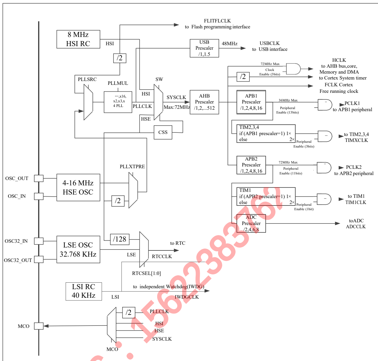
图 2 时钟树
