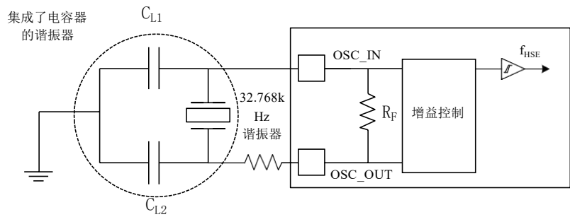
图 15 使用 32.768kHz 晶体的典型应用
