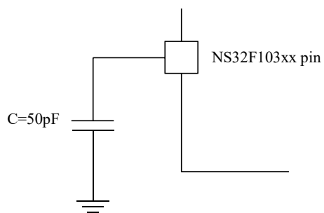
图 8 引脚的负载条件
