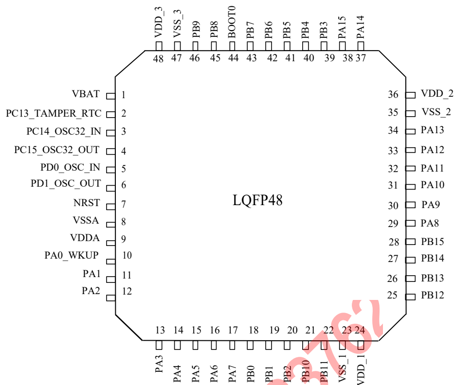
图 5 NS32F103xx 标准型 LQFP48 引脚分布
