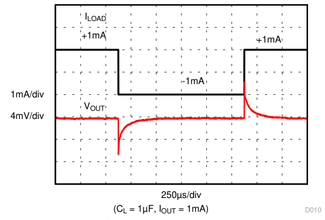
图 7-10. Load Transient
