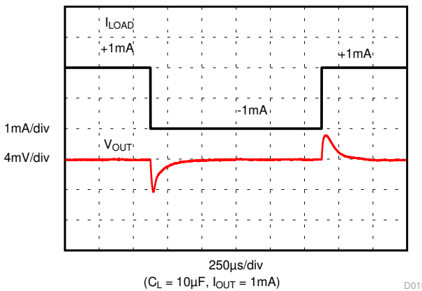
图 7-11. Load Transient
