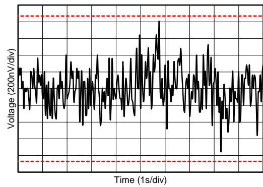
图 2. 0.1-Hz to 10-Hz Noise
