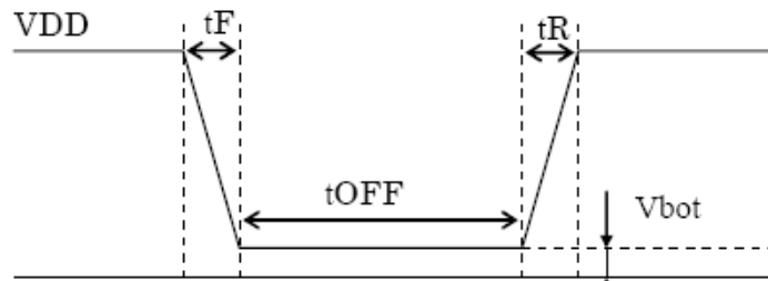
图 2、上升波形图
