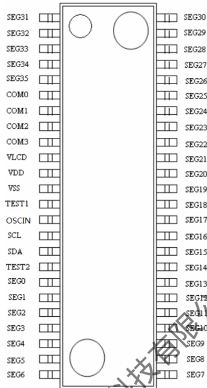
TSSOP48
