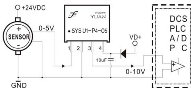
电压输入/电压输出 (V/V放大)
