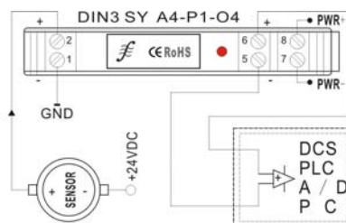
4-20mA 转 0-5V 接线图
