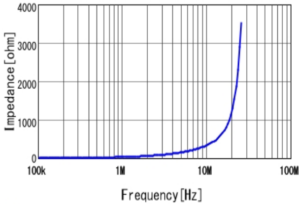
■ 1239AS-H-4R7M |Z|
