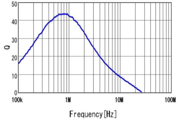
■ 1239AS-H-4R7M Q
