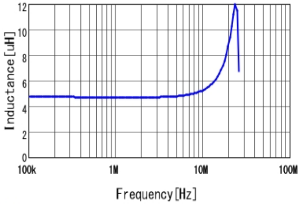
■ 1239AS-H-4R7M L
