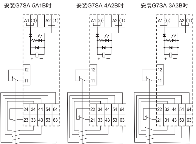
端子配置/内部连接图（顶视图）
