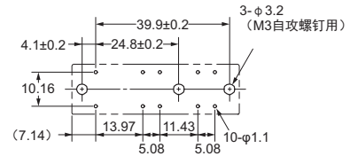
安装孔加工尺寸 (底视图) 尺寸公差为±0.1。
