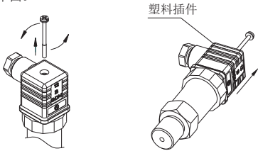
a) 旋出十字盘头 M3螺钉 图8-1
