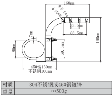
图9-4 安装支架尺寸图
