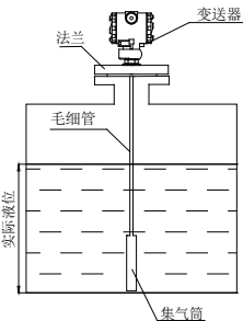
图9-2 法兰安装示意图
