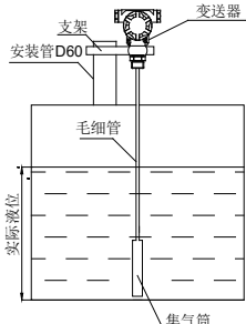
图9-1 支架安装示意图
