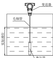
图9-3 螺纹安装示意图
