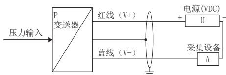
电流输出接线图8-4(两线制)
