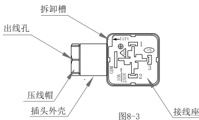
c) 用一字螺丝刀从拆卸槽插入撬出接线座。
