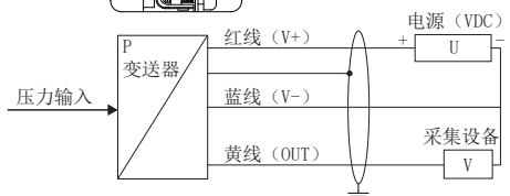
电压输出接线图8-5(三线制)
