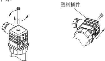
a) 旋出十字盘头 M3螺钉 图8-1 b) 按下图上所标注的塑料插件 图8-2
