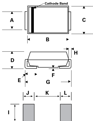
DO-214AC (SMA)
