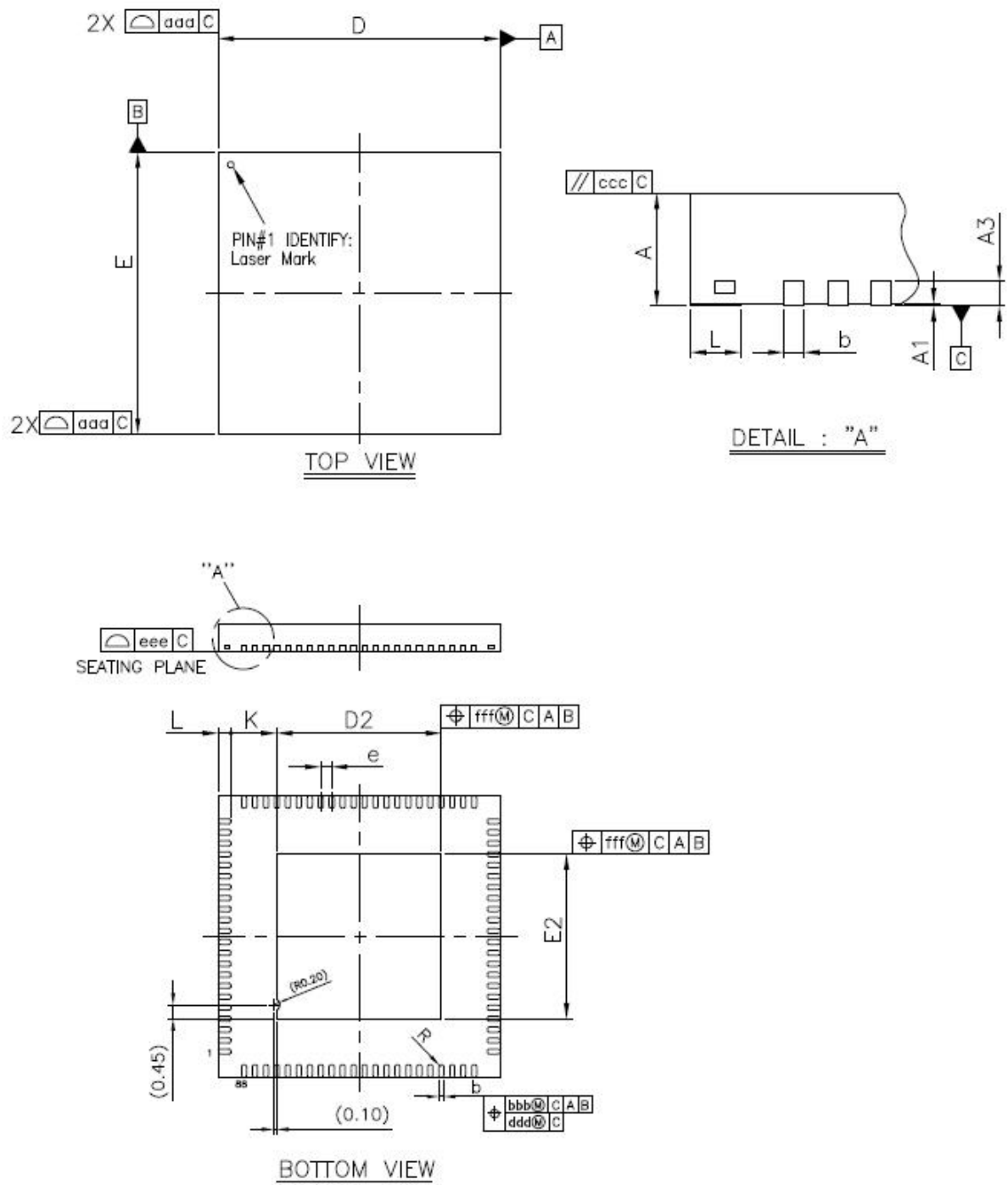
图 3-1 GK7205V200 芯片封装图
