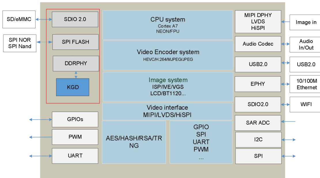
图 0-1: GK7205V200 功能框图
