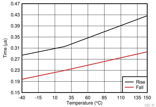
A. C_L=100\text{nF}
