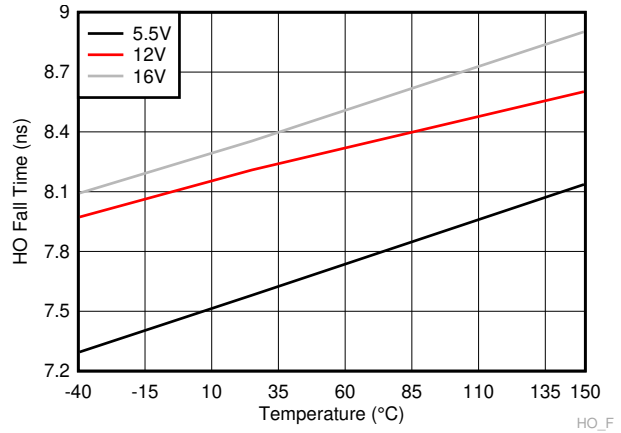
A. C_L=1800\text{pF}
