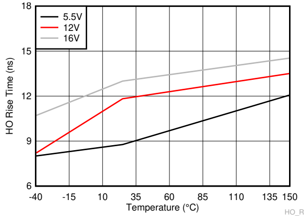
A. C_L=1800\text{pF}
