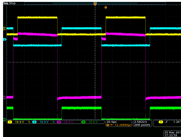
C_L = 1\text{ nF} Ch1 = HI Ch2 = LI Ch3 = HO Ch4 = LO
