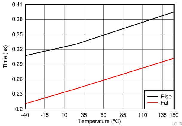
A. C_L=100\text{nF}
