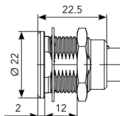
Front Mount (ER)
