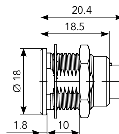
Front Mount (ER)
