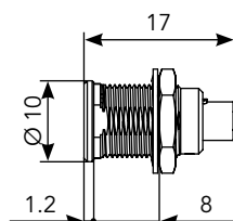
Front Mount (ER)
