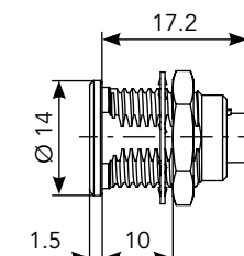
Front Mount (ER)
