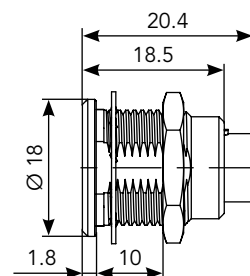
Front Mount (ER)
