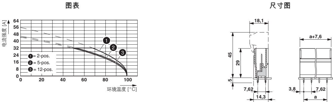
衰减曲线，用于：PC 5/...-ST1-7.62，带PCV 4/...-G-7.62 导体横截面：6 mm²
