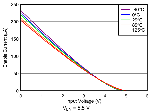
图 24. I_{EN} vs V_{IN}
