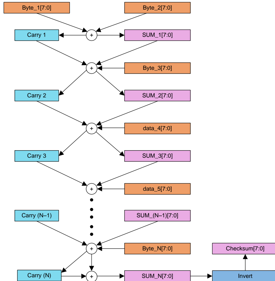
图 19. Checksum Calculation
