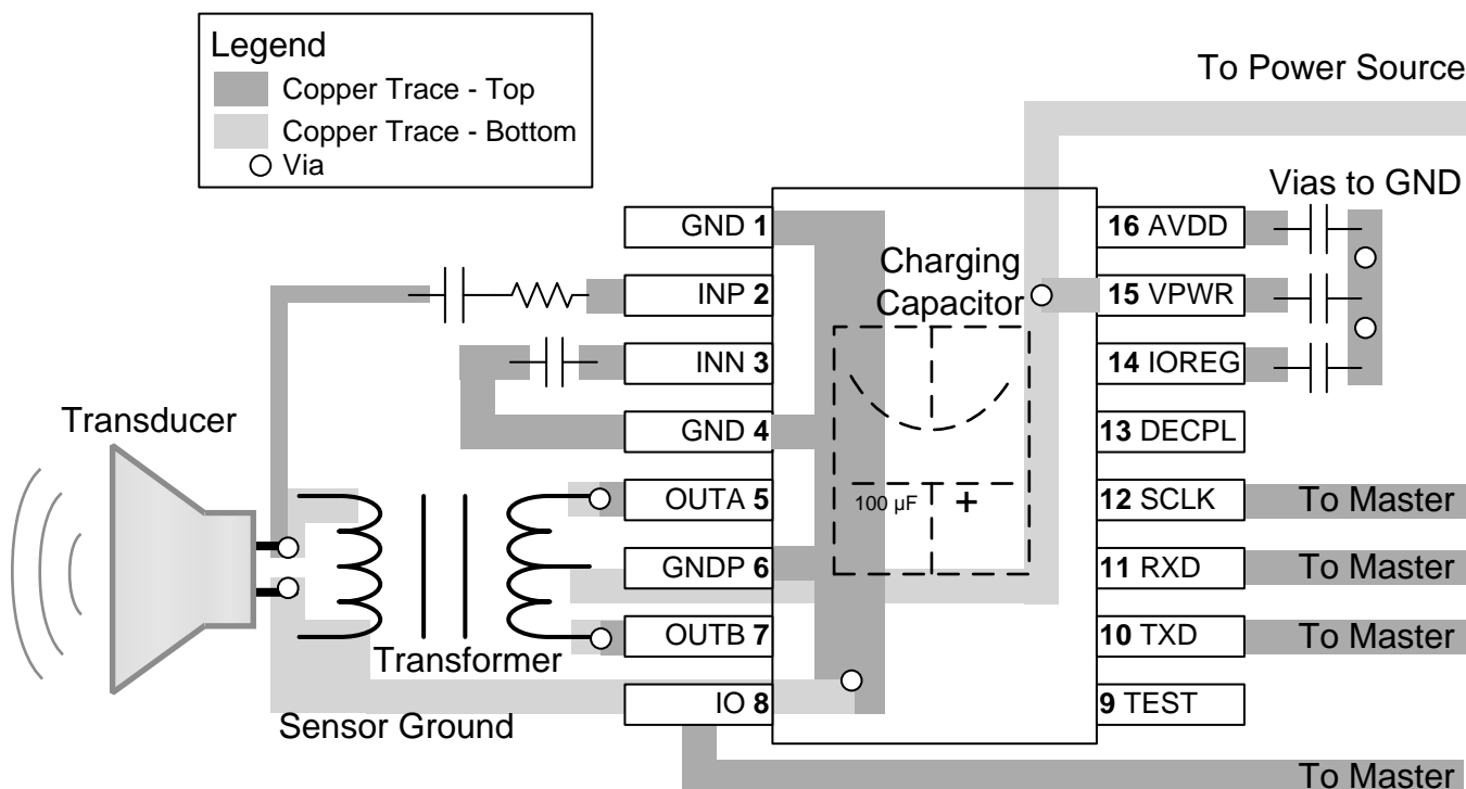
图 144. PGA460 Layout Example
