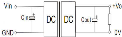
图 4 单路输出应用电路图
