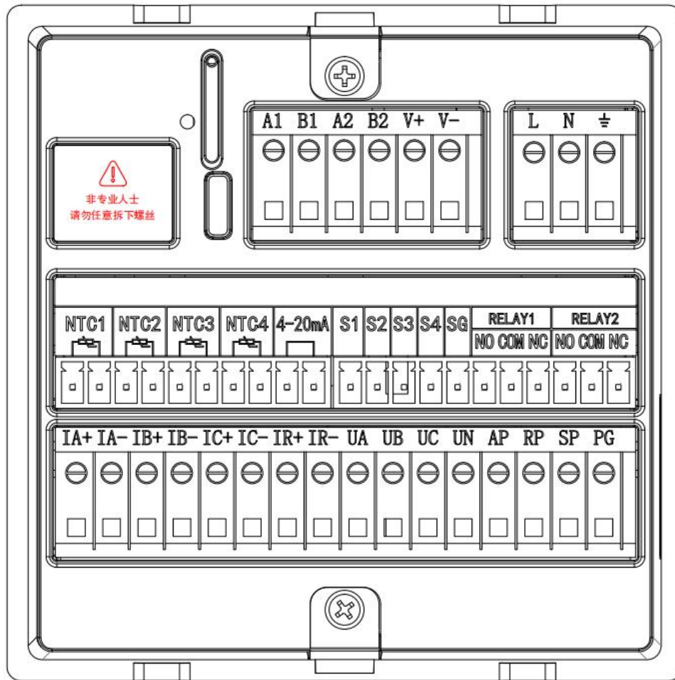
方式1 (3个CT): 三相四线的接线方式
