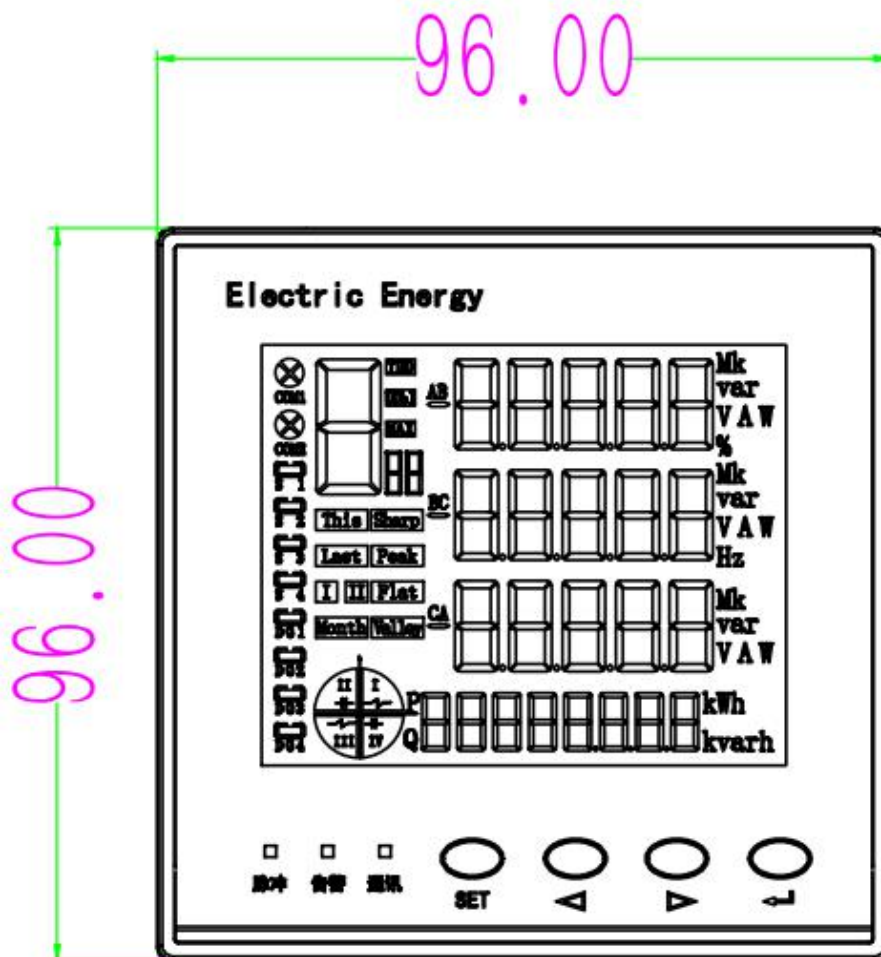
正面尺寸图
