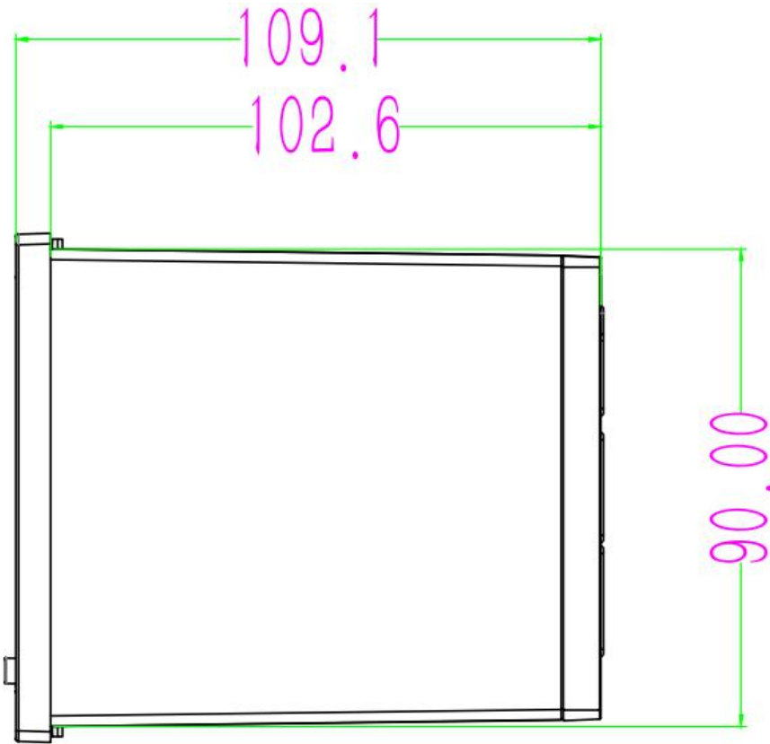
侧面尺寸图
