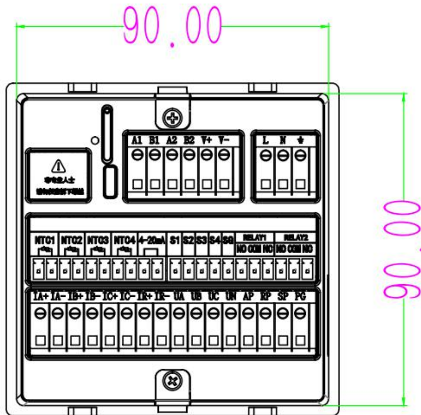
背面尺寸图
