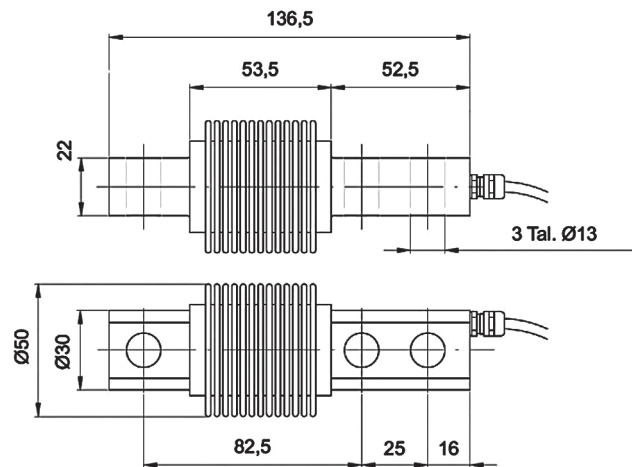
Dimensions in mm 尺寸为毫米
