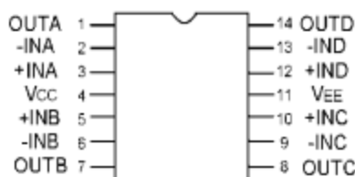
(D14S2·顶视图)
