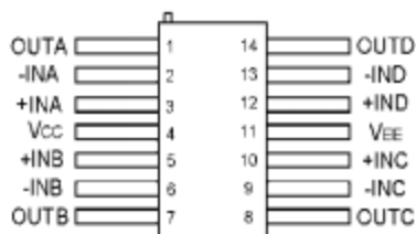
(F14-01·顶视图)
