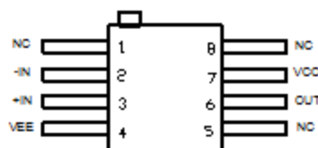
(F08-06·顶视图)
