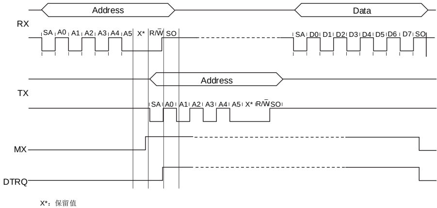
图 13 UART 写数据时序图
