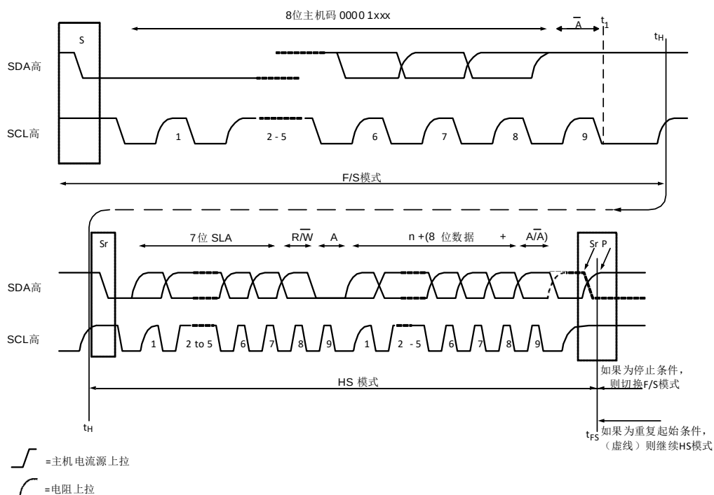
图 21 I²C 总线 HS 模式协议转换
