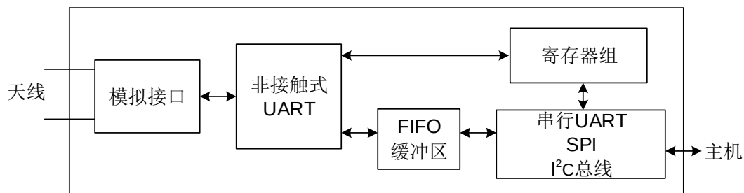
图 1 Si523 简化框图
