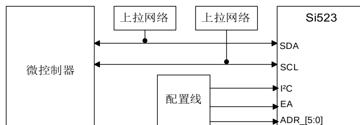
图 14 I 2 C 总线接口
