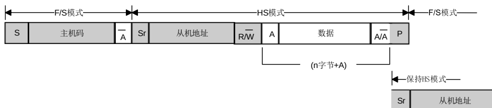
图 21 I²C 总线 HS 模式协议转换
