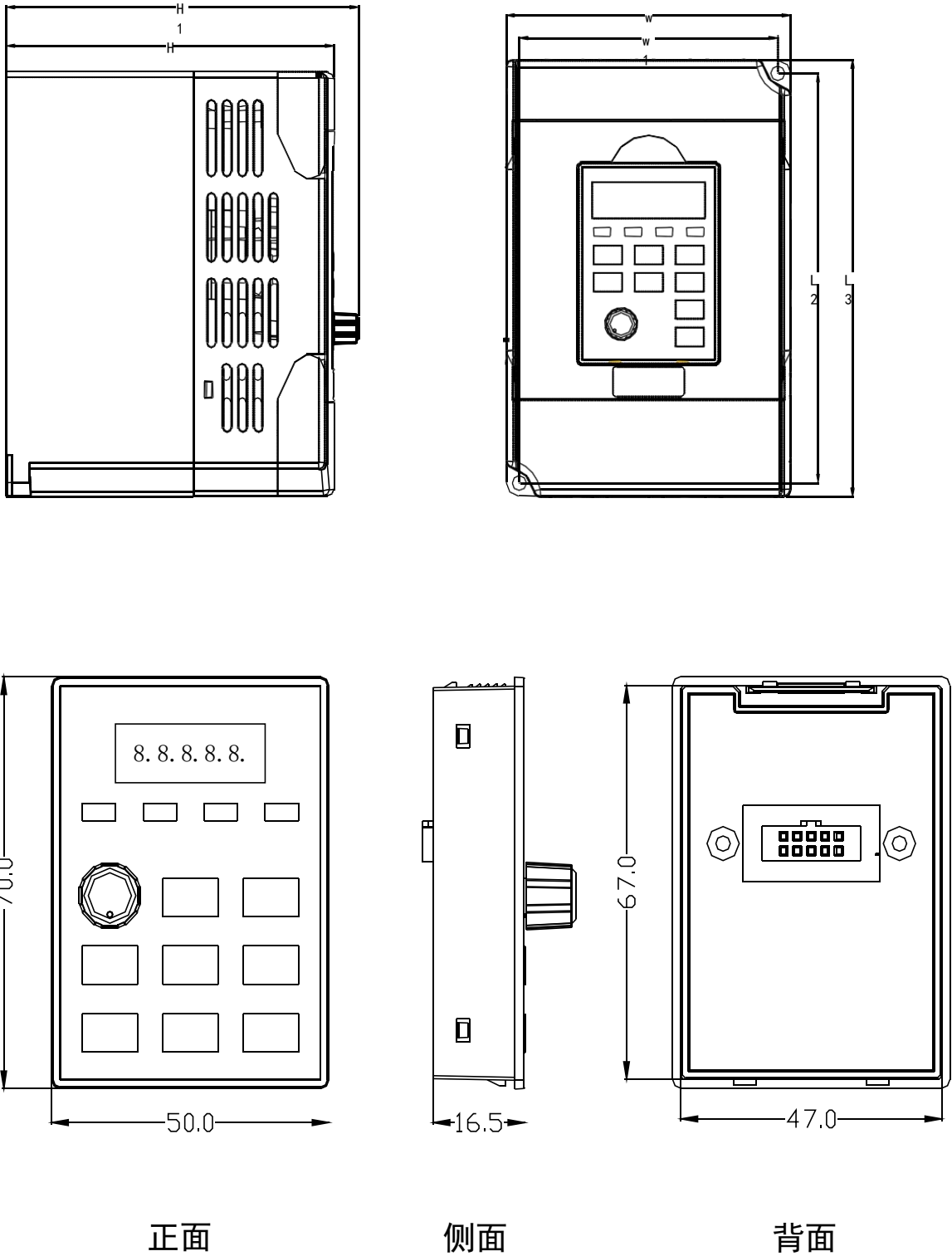
YP-A 面板尺寸图
