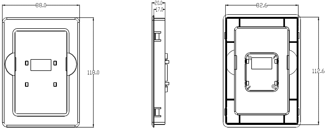
YP-D 托盘外形图(45KW 以上 键盘)
