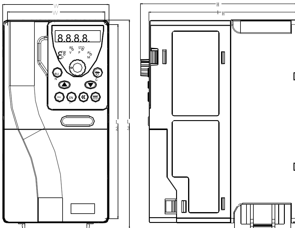
产品外形图
