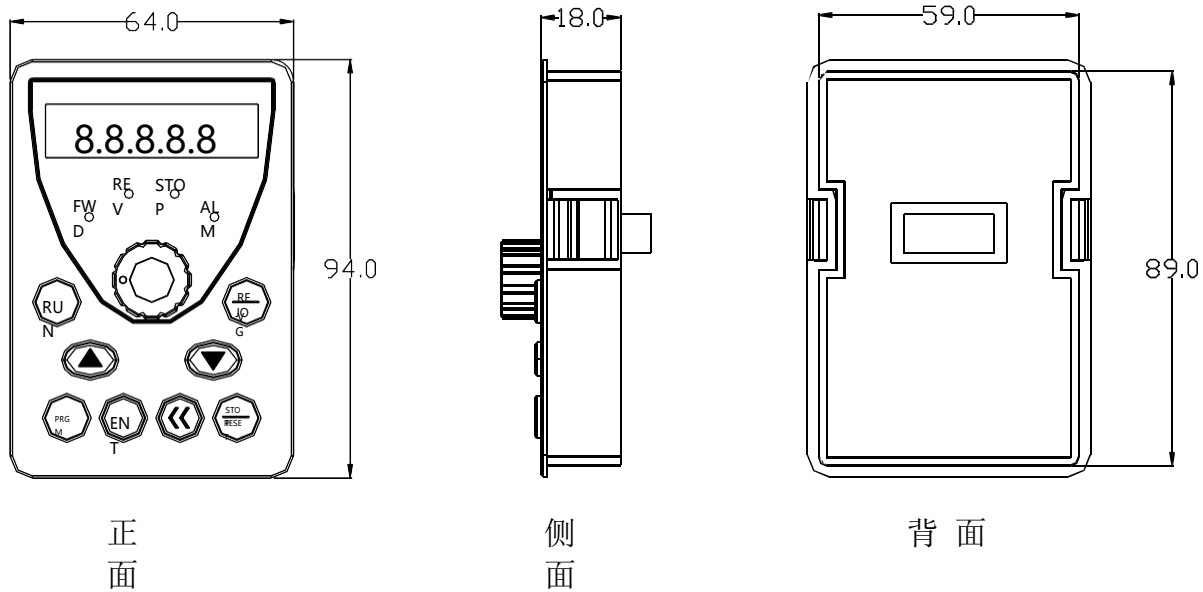
YP-C 面板尺寸图
