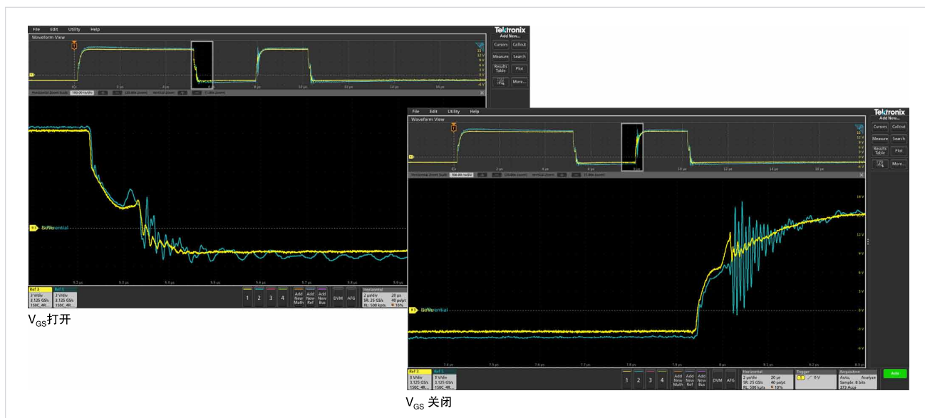
图 4. 差分探头 (蓝色轨迹) 与 IsoVu 光隔离探头 (黄色轨迹) 对比。
