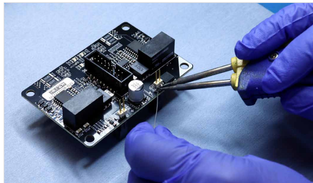
图 16. 经 V GS 节点焊接方针头部，测量高压侧栅极驱动信号。图片由 Wolfspeed 提供，获准重新印刷。
