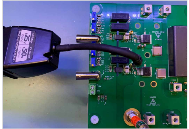
图 13. MMCX 连接器 - 实例 2。图片由 Wolfspeed 提供，获准重新印刷。
