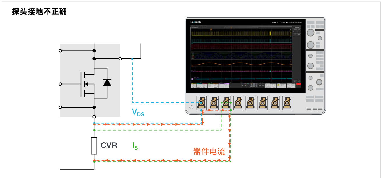
图 6. 在两只地电平参考探头连接到不同参考电压时，器件电流会旁路 CVR，流经地线和示波器。这会导致测量错误，并可能会导致设备损坏。
