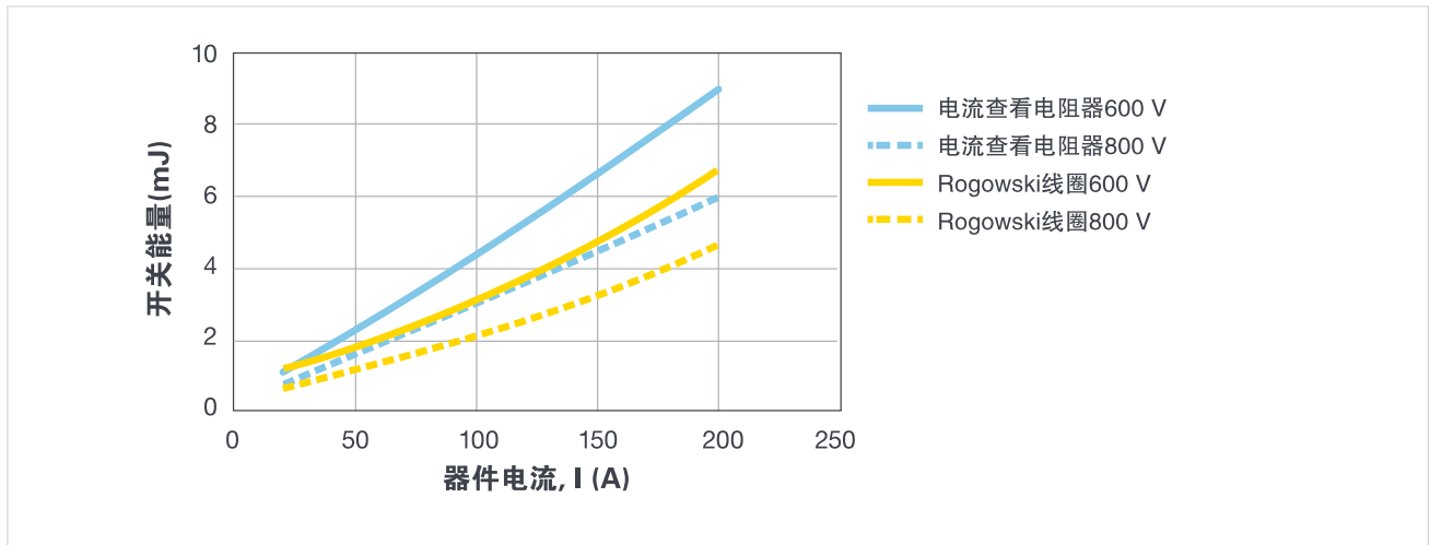
图 10. 使用不同探头 (CAB011M12FM3, T_J = 150^{\circ}\text{C} , R_G = 1\Omega ) 估算开关损耗 ( E_{\text{off}} + E_{\text{on}} )。
