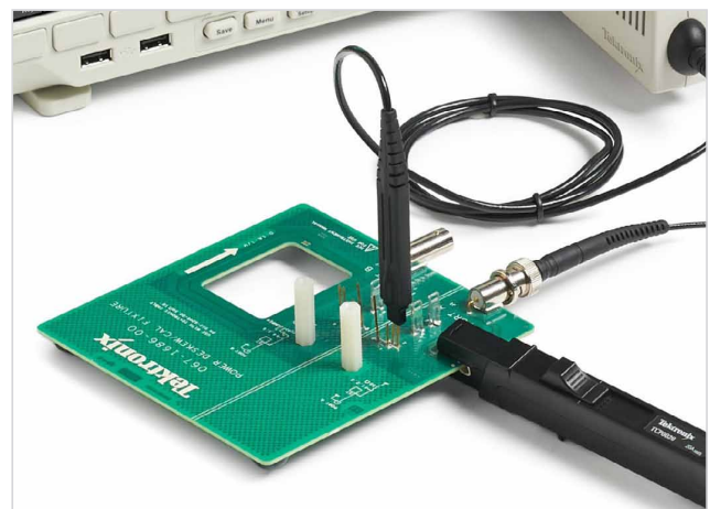
图 11. 功率测量时延校正和校准夹具 (067-1686-00)。这些连接装置提供了一种方便的方式，可以补偿电压探头和电流探头之间的时延。
