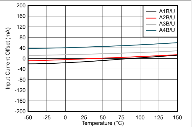
图 7-2. TMCS1108-Q1 Input Offset Current vs. Temperature
