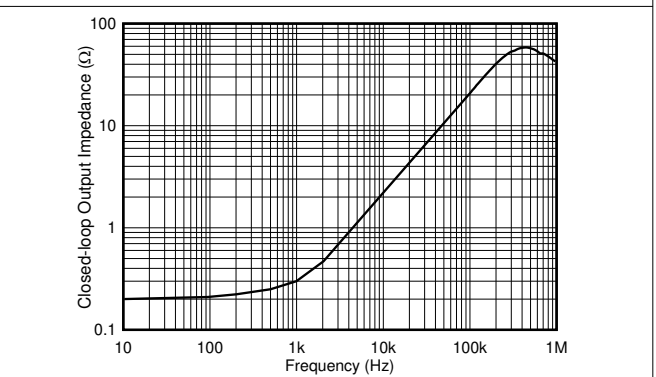
图 7-6. Output Impedance vs. Frequency
