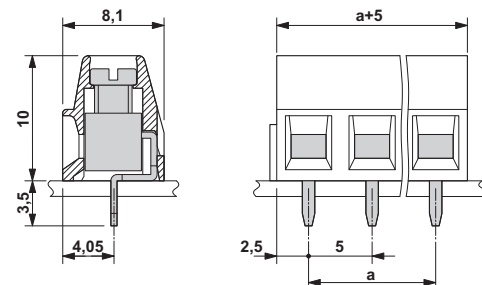
尺寸图
