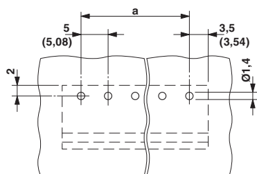
钻孔图
