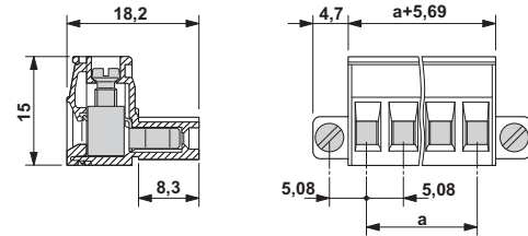
尺寸图
