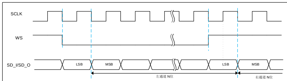
图 6-58 philips 数据格式
