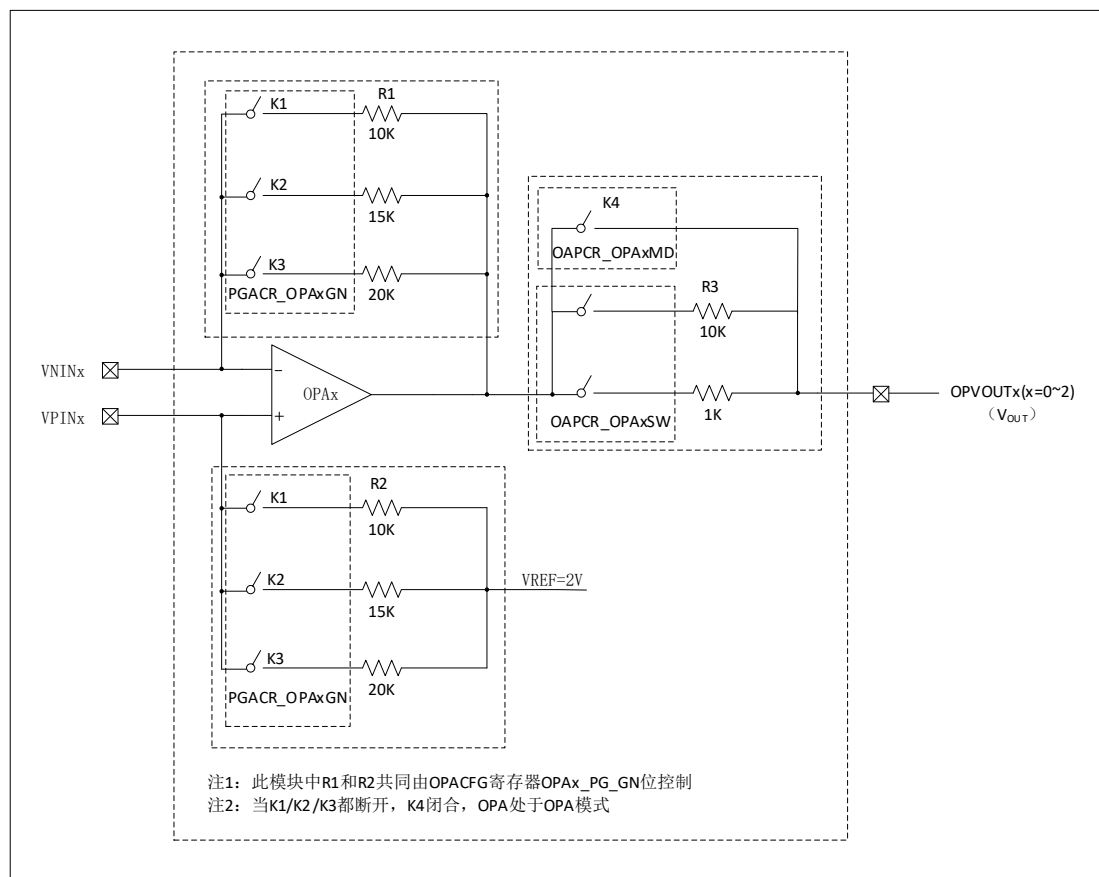
图 6-95 放大器框图
