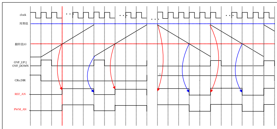
图 6-75 边沿对齐模式下 PWM 信号产生波形
