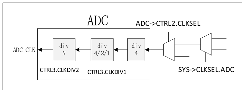
图 6-86 ADC 时钟示意图
