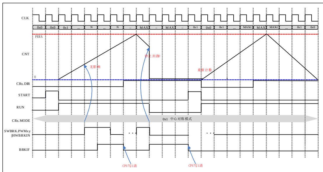
图 6-73 硬件刹车控制和软件刹车控制计数器计数情况
