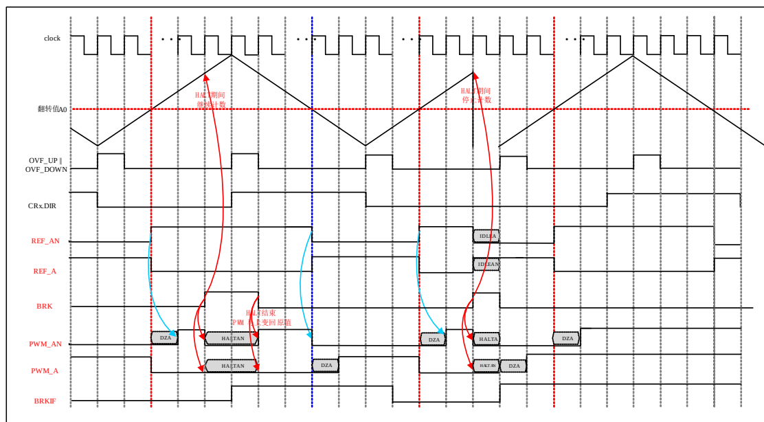
图 6-78 BRK 中心对齐模式下 PWM 信号产生波形
