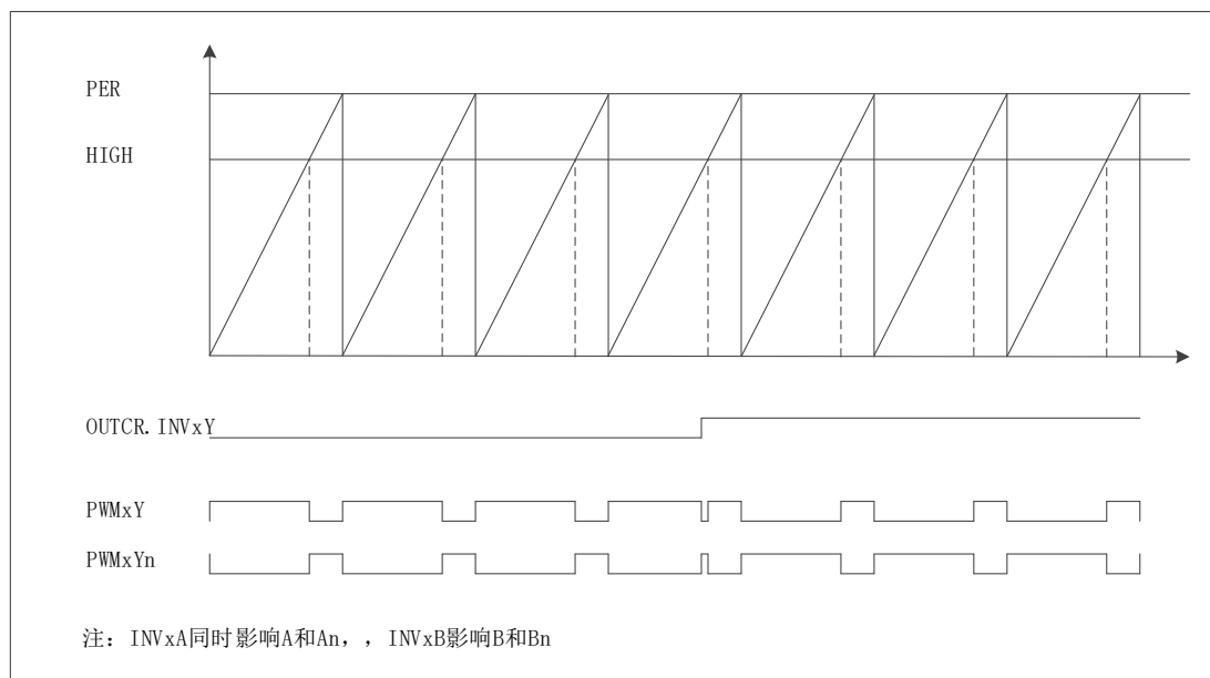
图 6-82 电平翻转示意图
