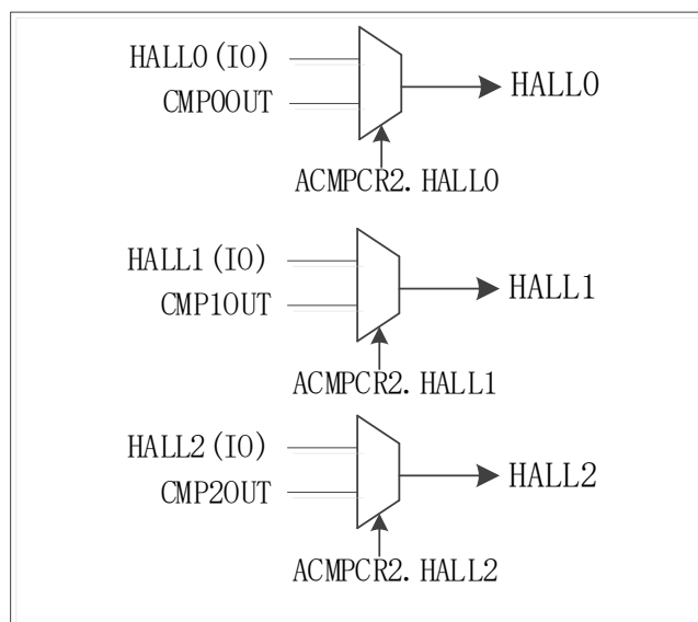
图 6-92 HALL 对应关系图
