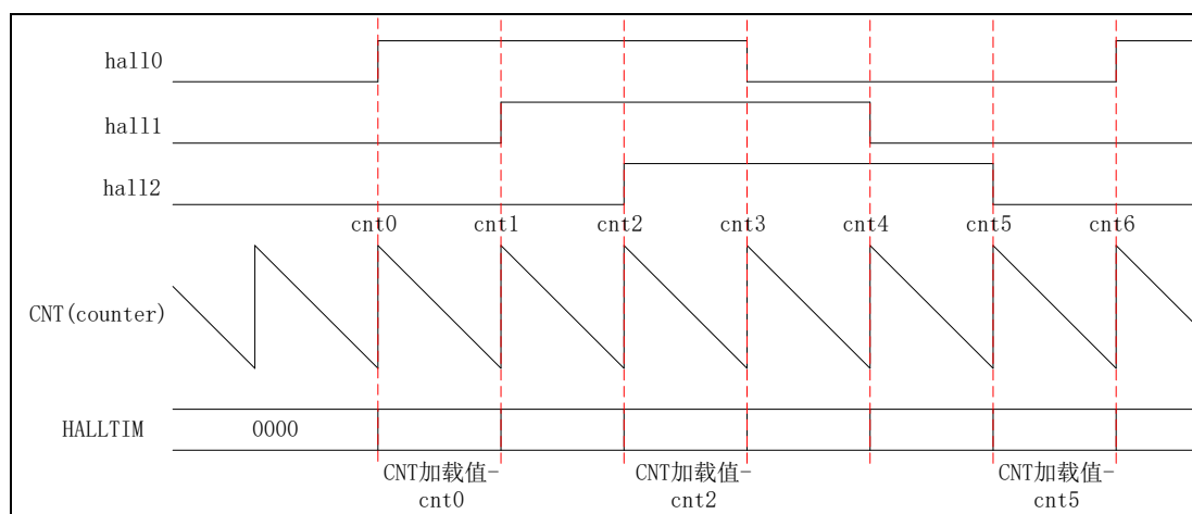
图 6-18 HALL 记录值
