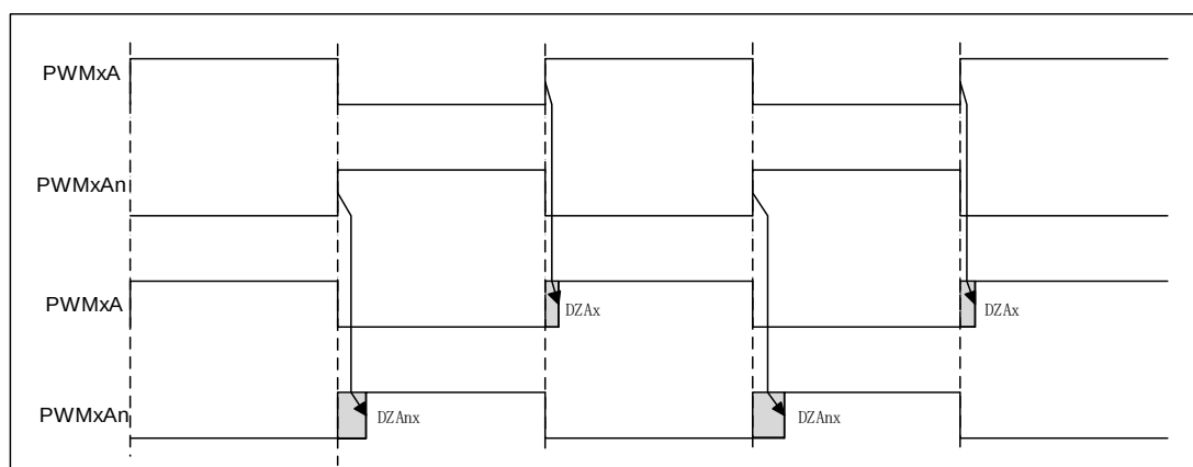
图 6-66 PWM 死区示意图
