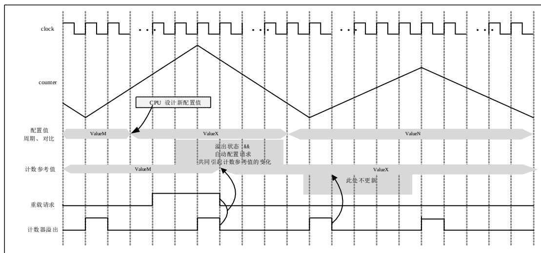
图 6-74 计数器重载波形
