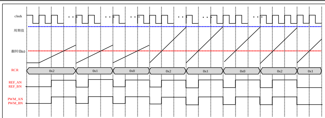
图 6-80 重复计数功能波形图
