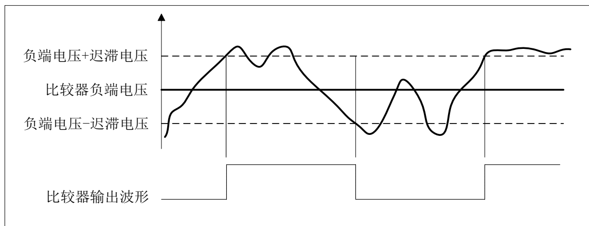
图 6-91 比较器迟滞功能示意图
