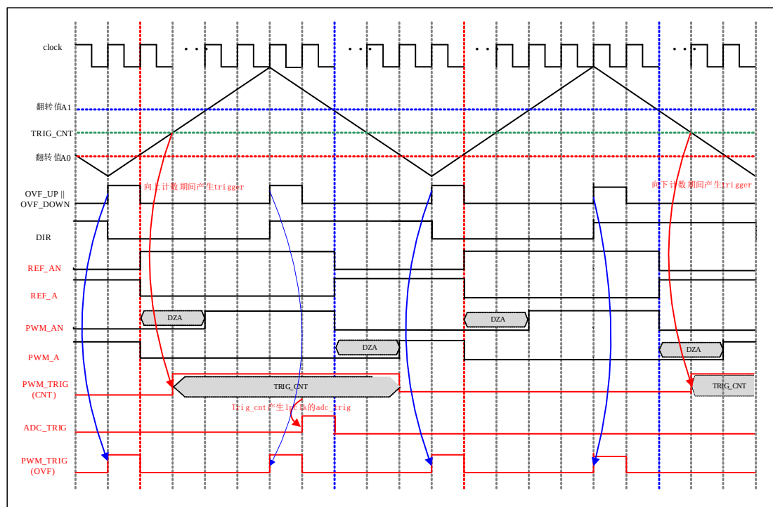
图 6-79 TRIGGER 控制波形
