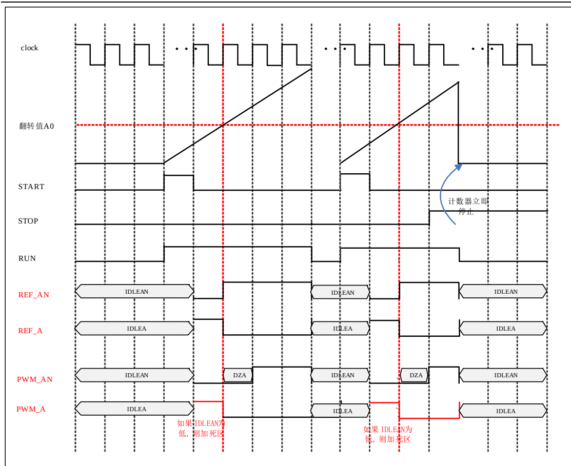
图 6-67 边沿对齐模式下向上计数计数器启动与停止波形
