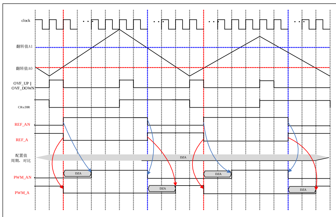
图 6-77 非对称中心对齐模式下 PWM 信号产生波形
