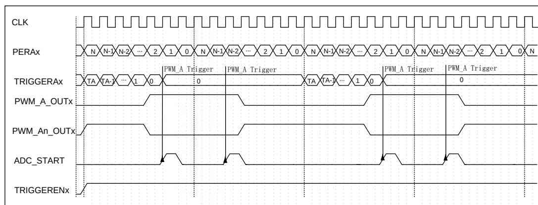
图 6-87 中心对称模式下 PWM 触发 ADC 采样示意图
