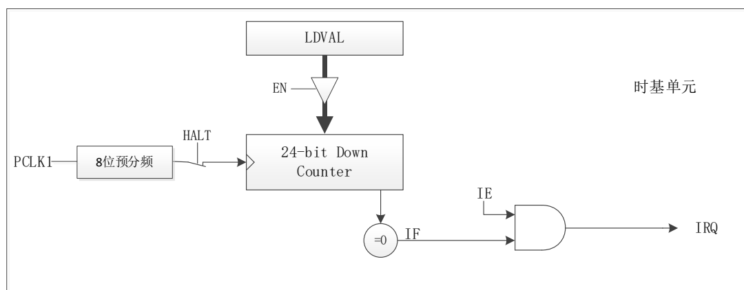
图 6-20 BTIMER 模块结构框图
