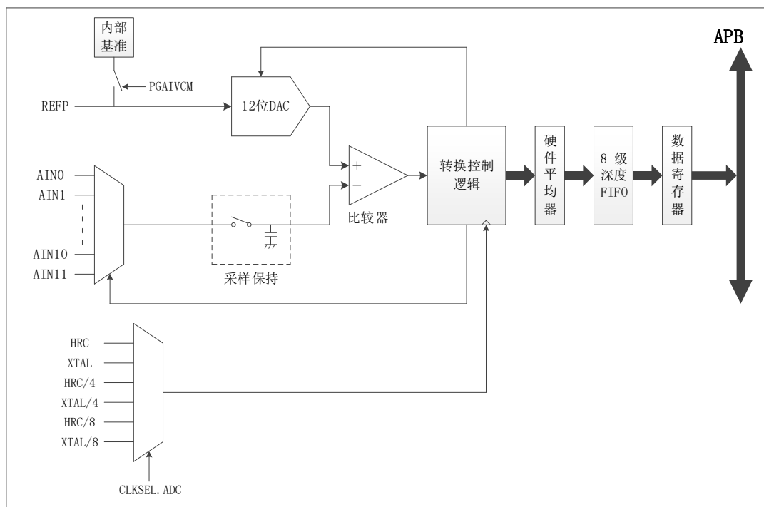
图 6-85 ADC 模块结构框图
