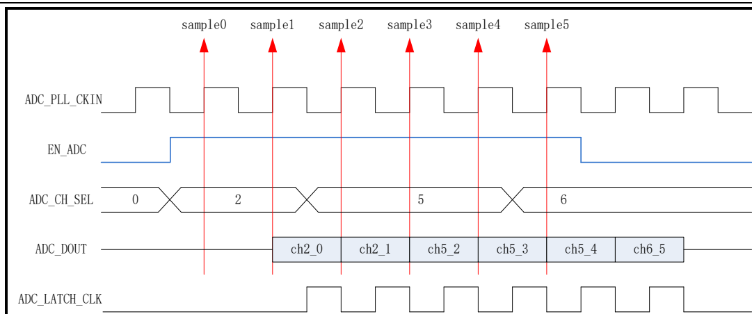
图 6-89 SAR ADC 多通道连续采样示意图
