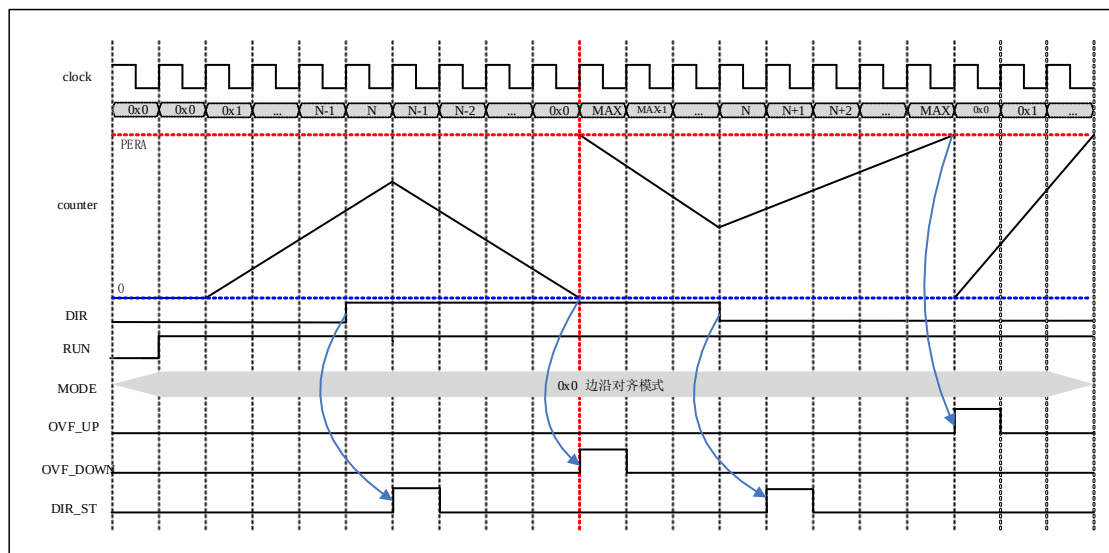
图 6-71 边沿对齐模式下计数器计数过程波形
