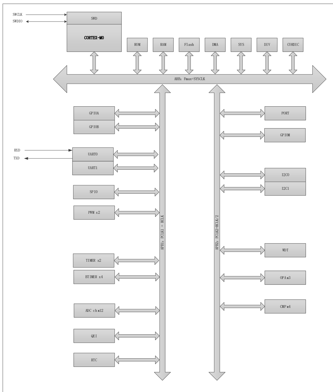
图 4-1 功能方框图
