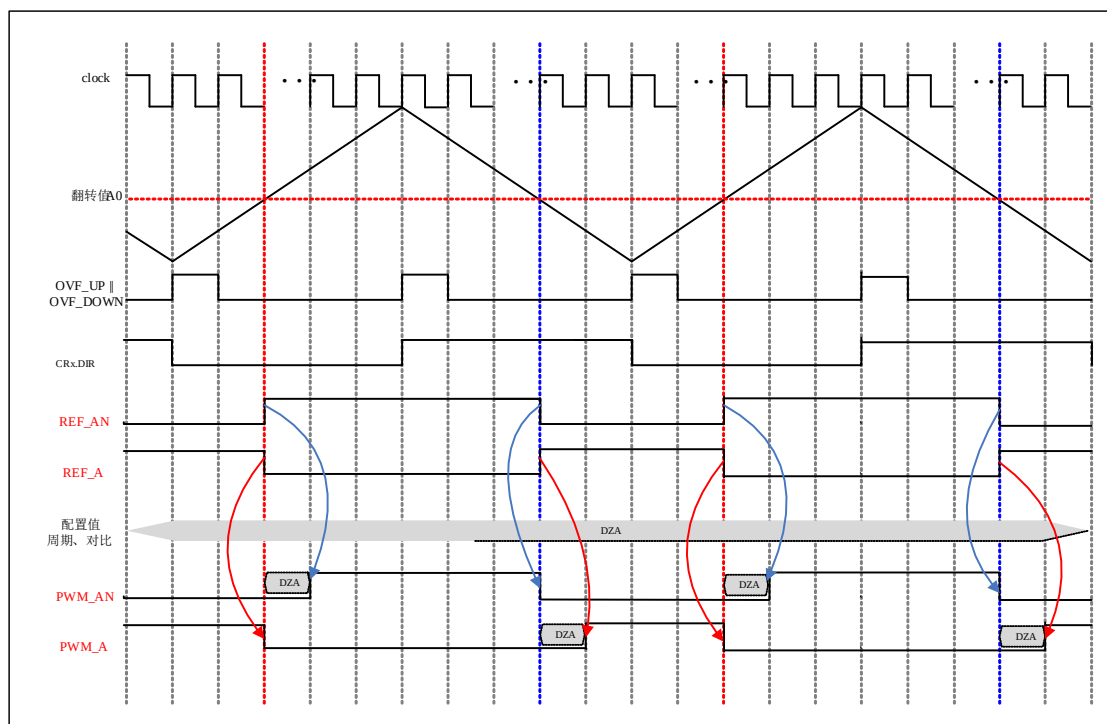
图 6-76 中心对齐模式下 PWM 信号产生波形
