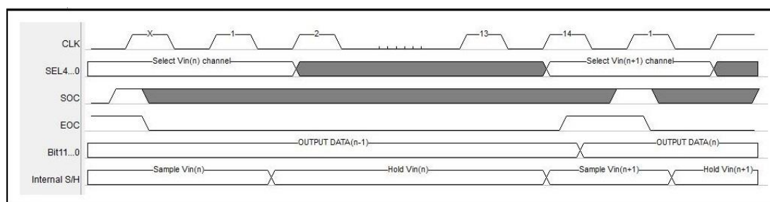
图 6-88 SAR ADC 连续采样示意图
