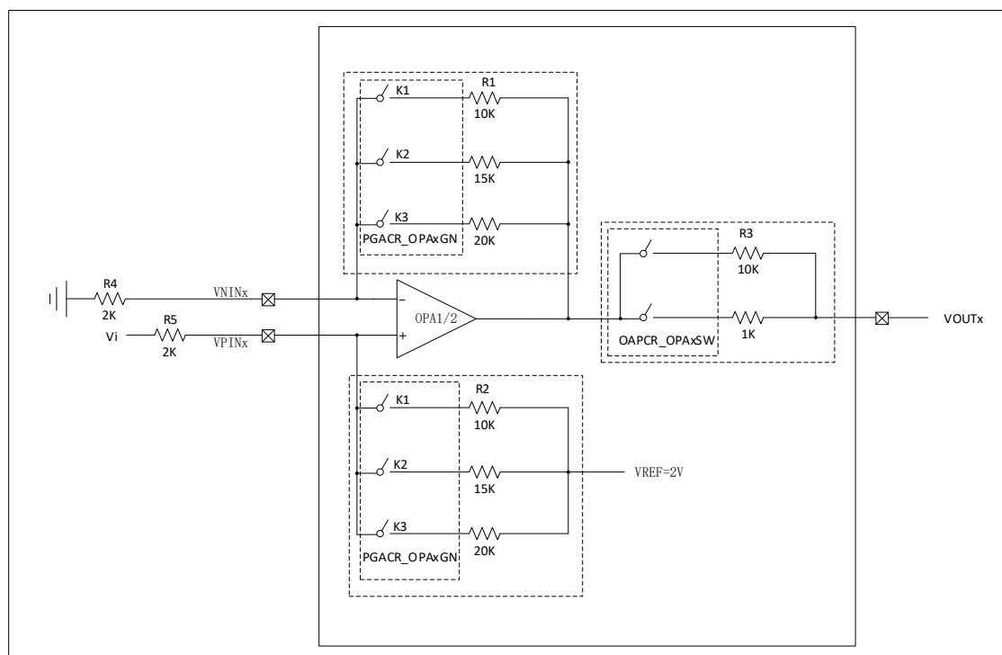
图 6-98 PGA 应用参考图
