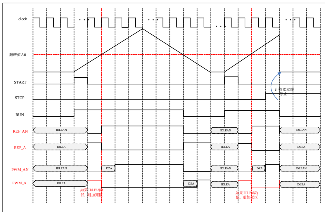
图 6-69 中心对齐模式下计数器启动与停止波形
