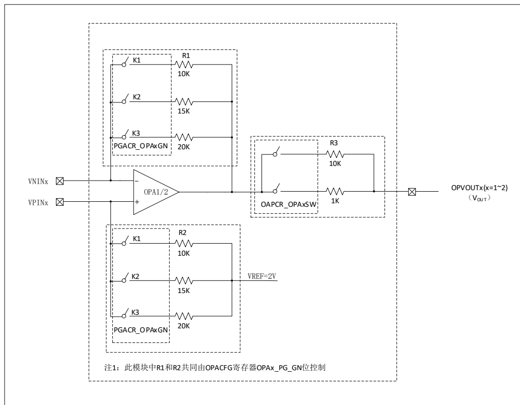
图 6-97 PGA 内部结构图
