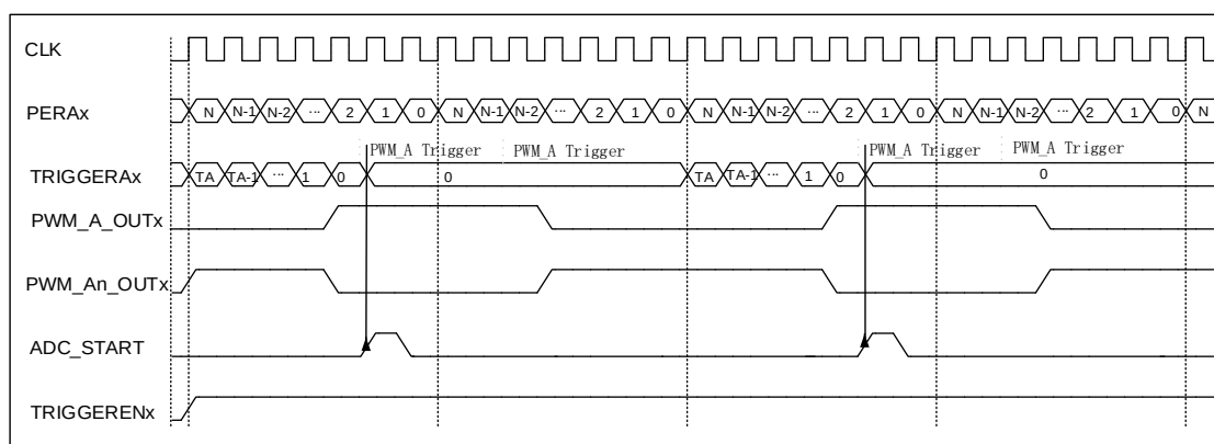
图 6-81 PWM 触发 ADC 采样示意图
