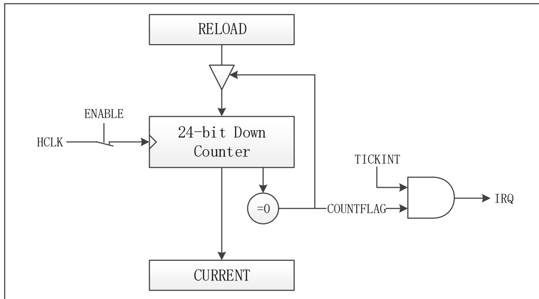
图 6-1 systic 模块结构图
