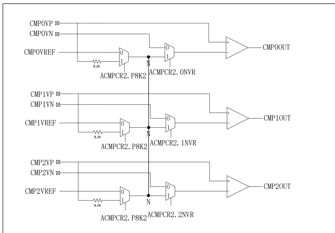
图 6-94 P 端分压模式结构图
