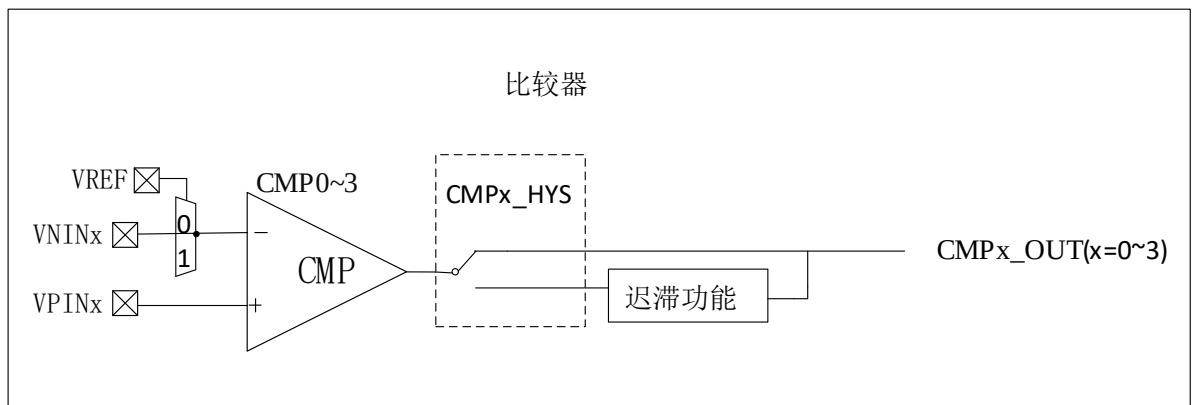
图 6-90 比较器框图
