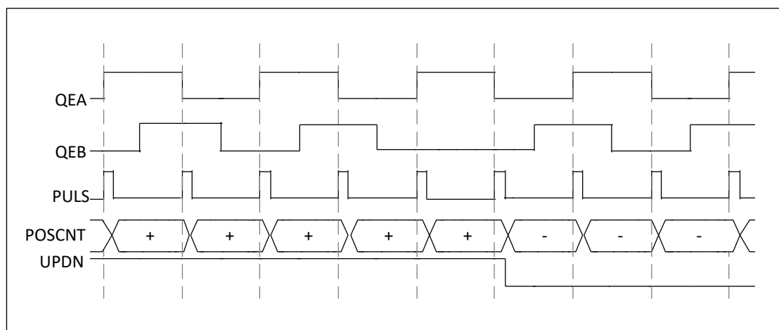
图 6-29 正交编码器 x2 计数模式示意图
