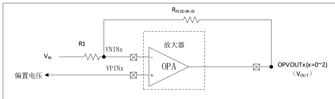
图 6-96 典型放大电路
