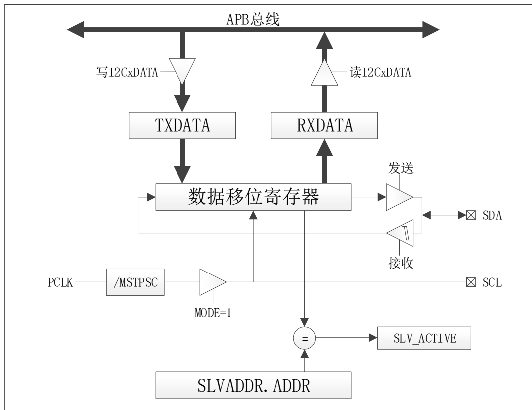
图 6-47 I2C 模块结构框图
