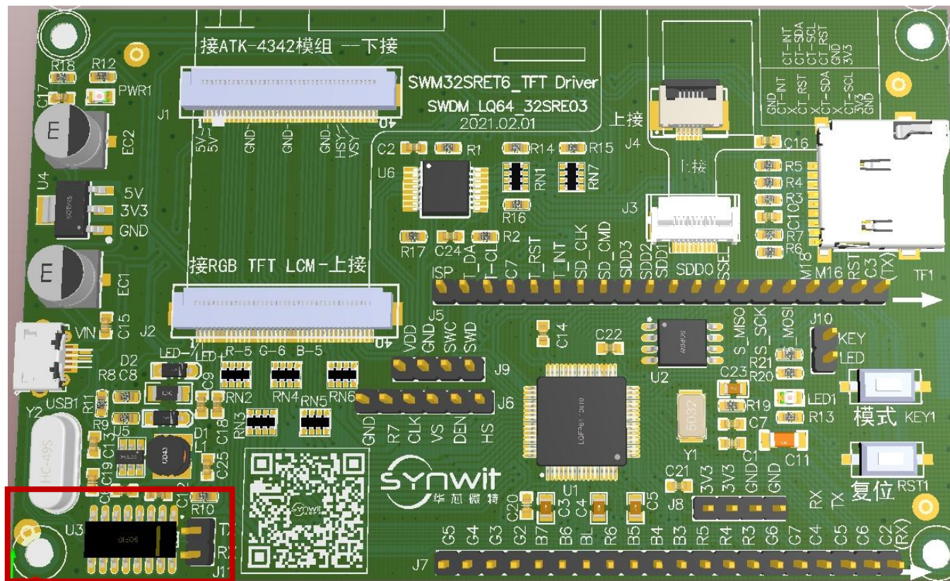
SWM32SRET6-50 RE03 最小系统板板框预览图
