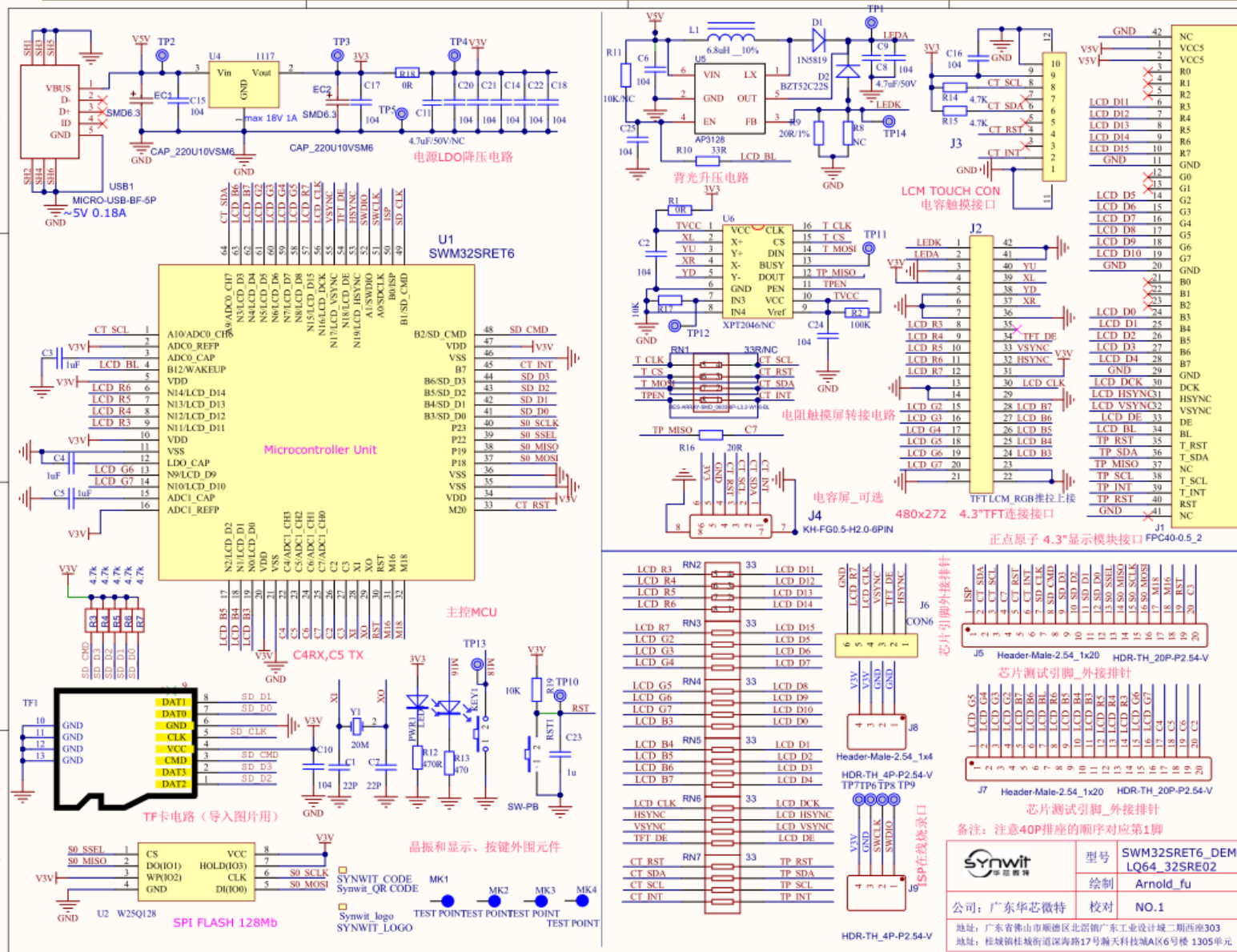
SWM32SRET6-50 RE02 最小系统板原理图
