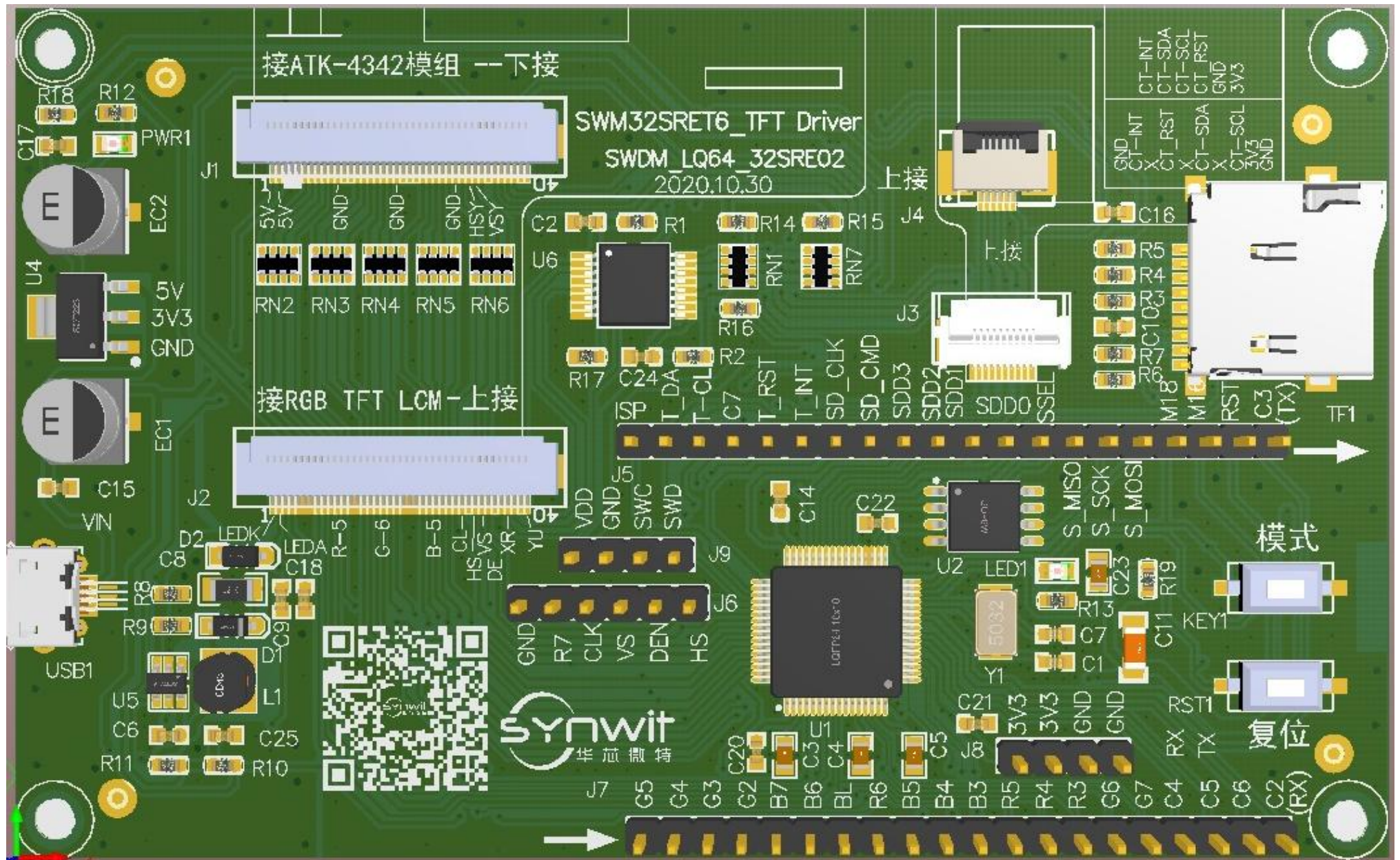
SWM32SRET6-50 RE02 最小系统板板框预览图
