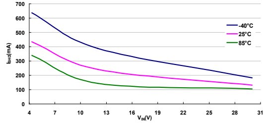
Iq VS VIN
