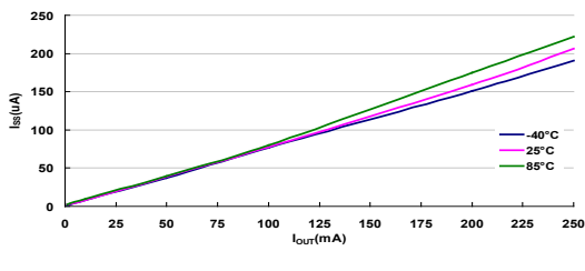
I_{SS} vs I_{OUT} : HT7350-7 ( V_{IN}=7.0V )
