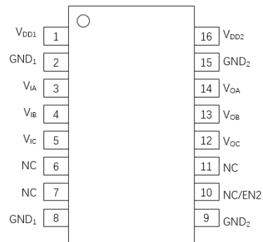
图 3. π130Uxx 管脚定义
