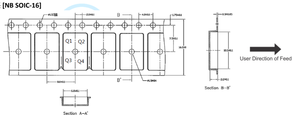
图 20. 16 引脚窄体 SOIC 封装 [NB SOIC-16] 包装信息-尺寸单位(mm)
