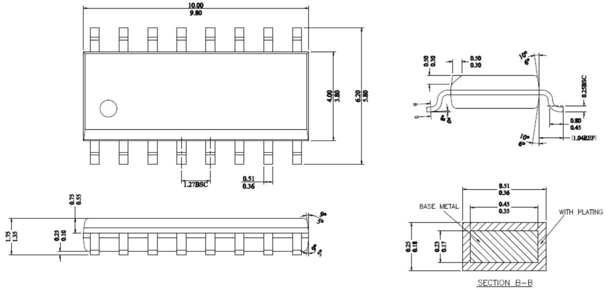
图 13. NB SOIC-16 封装外形尺寸-尺寸单位(mm)
