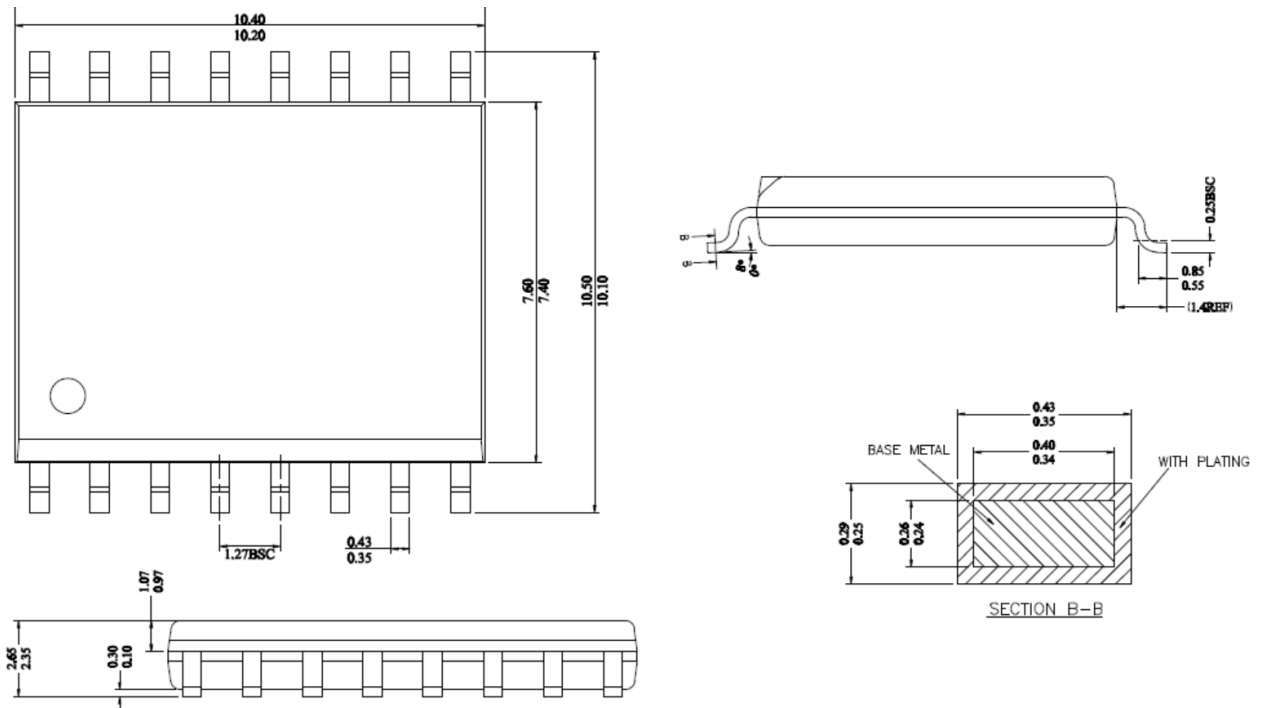
图 14. WB SOIC-16 封装外形尺寸-尺寸单位(mm)
