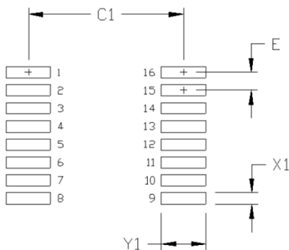
图 18. 16 引脚 SSOIC 封装 [16-Lead SSOP] 焊盘图案
