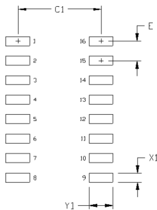
图 16. 16 引脚窄体 SOIC 封装 [NB SOIC-16] 焊盘图案
