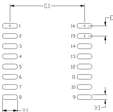
图 17. 16 引脚宽体 SOIC 封装 [WB SOIC-16] 焊盘图案
