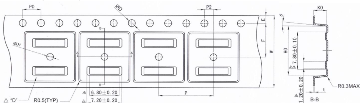
图 20. 16 引脚窄体 SOIC 封装 [NB SOIC-16] 包装信息-尺寸单位(mm)
