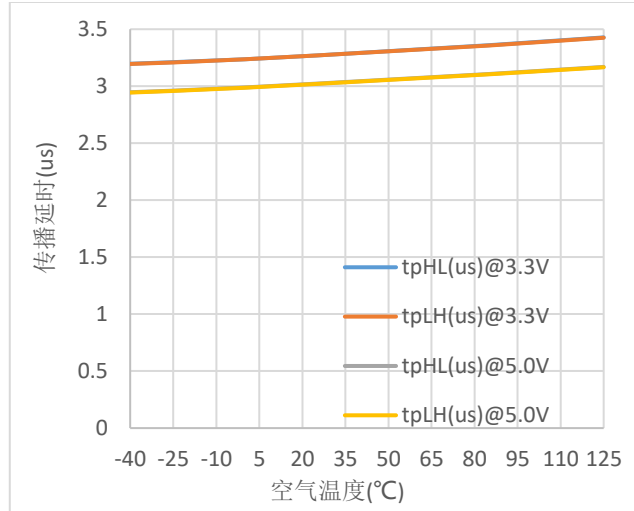
图 7. \pi 13xU3x 传输延时 vs. 空气温度
