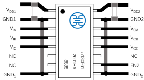
图 11. 推荐的印刷电路板布局
