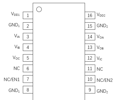
图 4. π131Uxx 管脚定义
