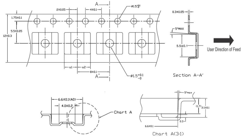
图 22. 16 引脚宽体 SSOP 封装包装信息-尺寸单位(mm)
