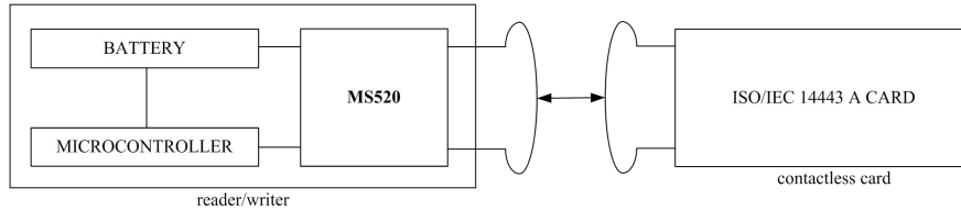
图 4. MS520 读写模式
