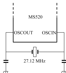
图 10. 石英晶体的连接
