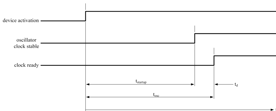
图 11. 振荡器起振时间
