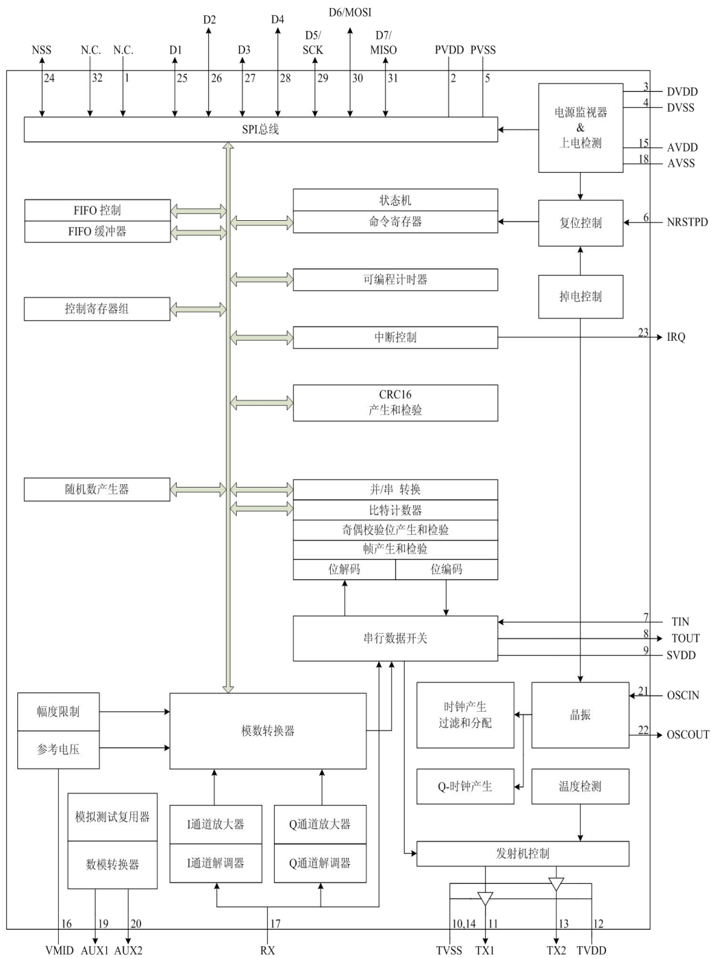
图1. MS520内部框图
