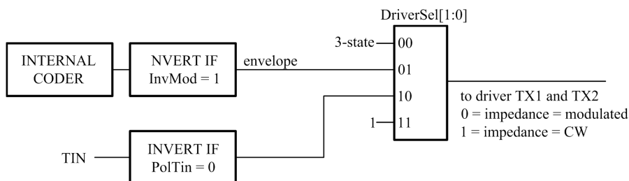
图 8. TX1 和 TX2 的串行数据转换
