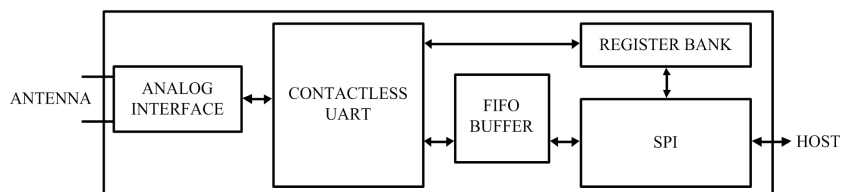
图 2. 简化的 MS520 框图
