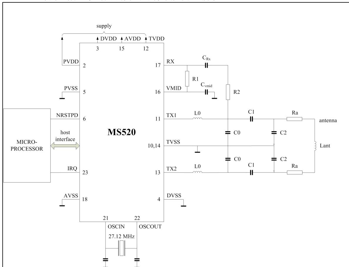
图 15. 典型应用图
