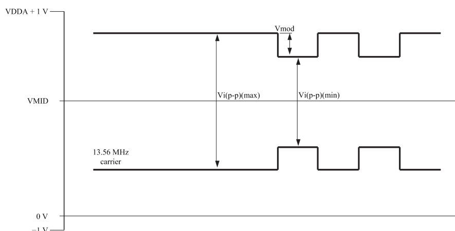
图 12. 管脚 RX 输入电压范围
