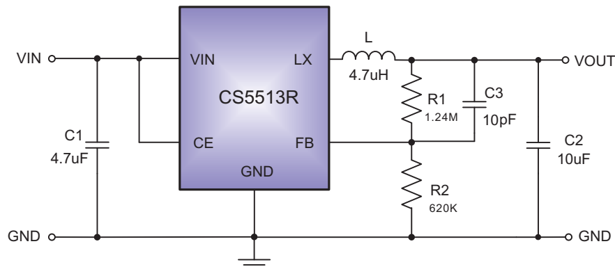
图1.应用图
