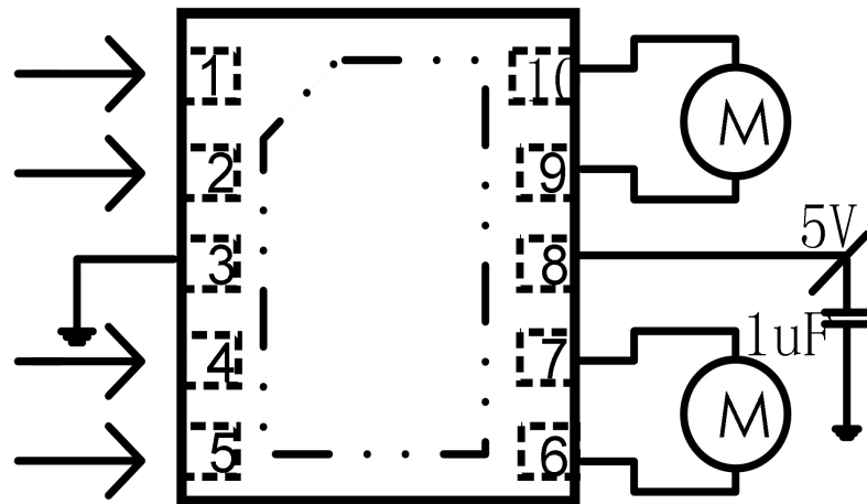
应用图：驱动两个直流电机
