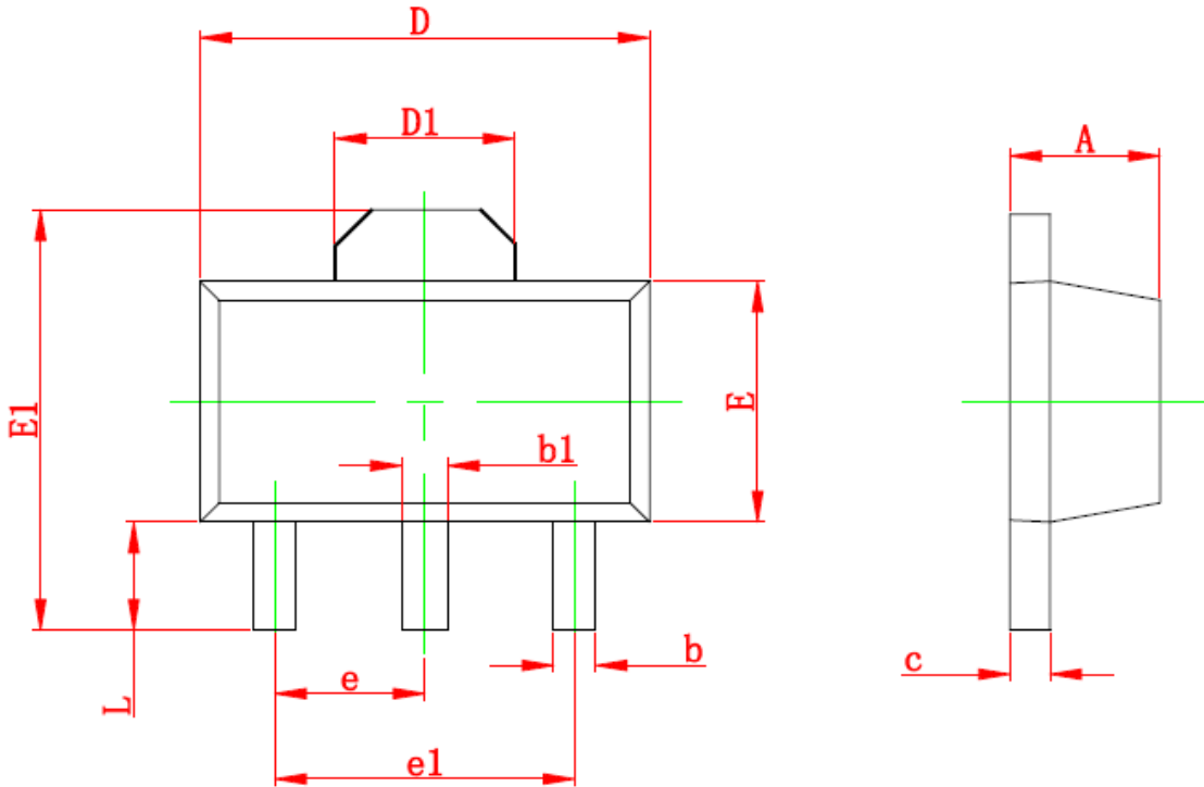
SOT89-3 封装尺寸图:
