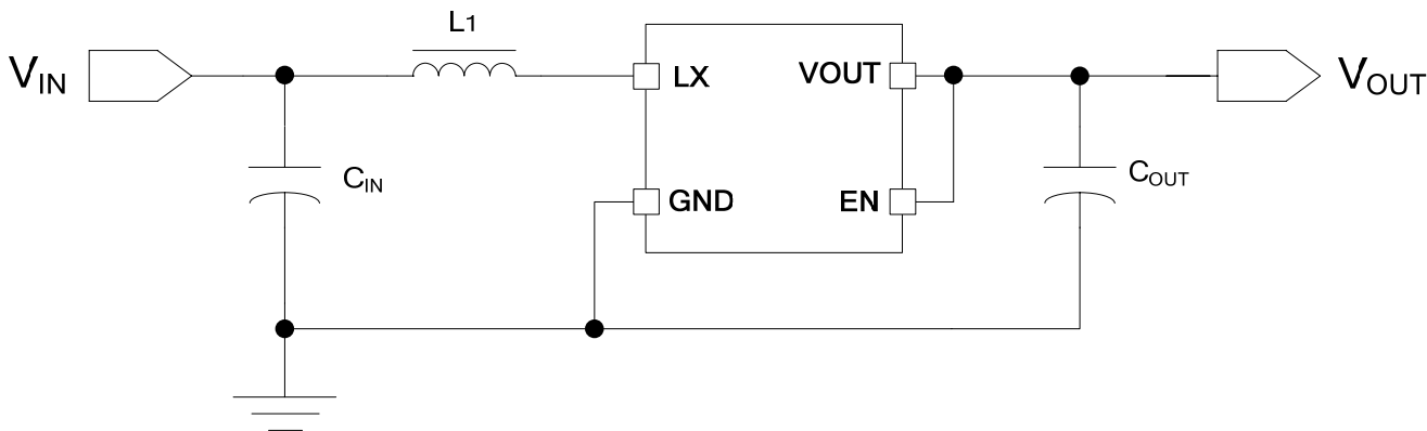
图 1：FS2112 典型应用电路图
