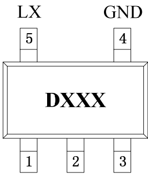
EN VOUT NC FS2112AXXB (SOT23-5)
