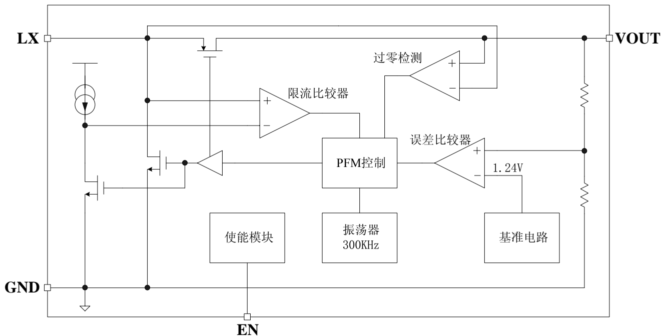
图 2: FS2112 的内部电路方框图
