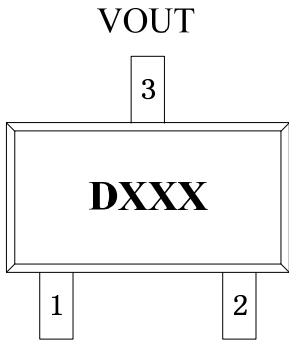
GND LX FS2112AXXA (SOT23)
