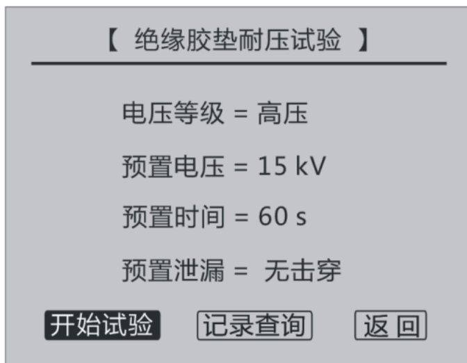
图 3.8 绝缘胶垫界面
