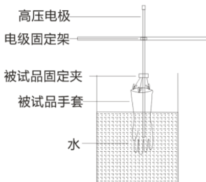
图 4.3 绝缘手套试验示意图
