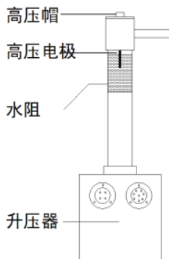
图 4.1 水电阻安装示意图
