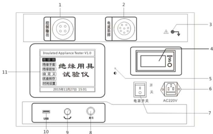
图 1.1 绝缘靴（手套）操作箱面板结构图
