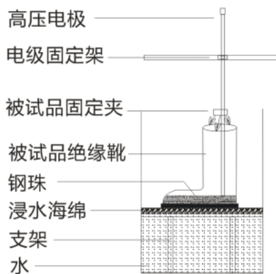
图 4.2 绝缘靴试验示意图
