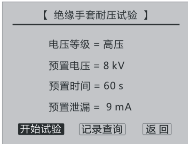
图 3.7 绝缘手套界面
