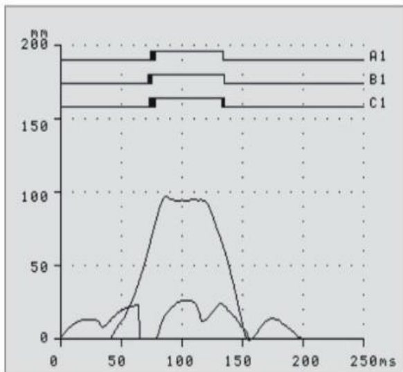
合--分闸测试图形
