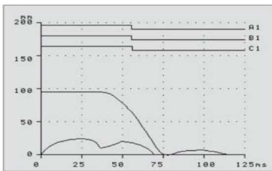
分闸测试图形
