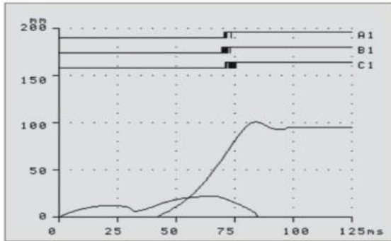
合闸测试图形
