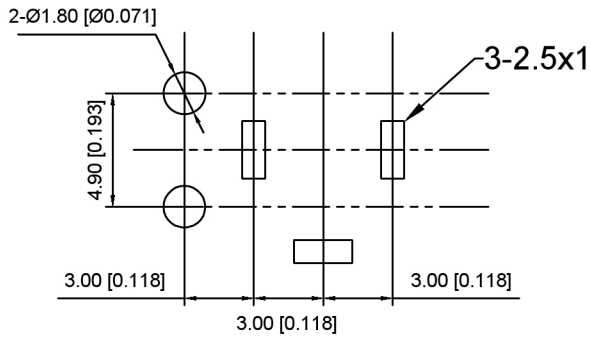
线路板开孔尺寸 P.C.B LAYOUT
