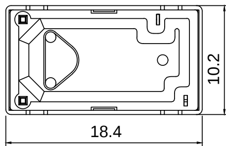
底视图
