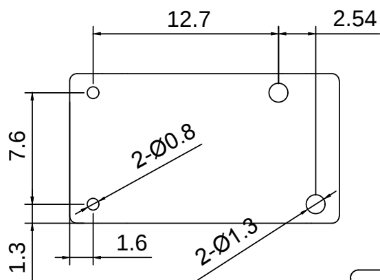
PCB布局 (底视图)
