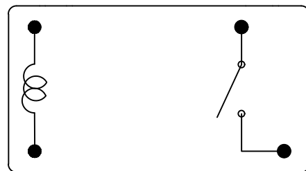
接线图 (底视图)
