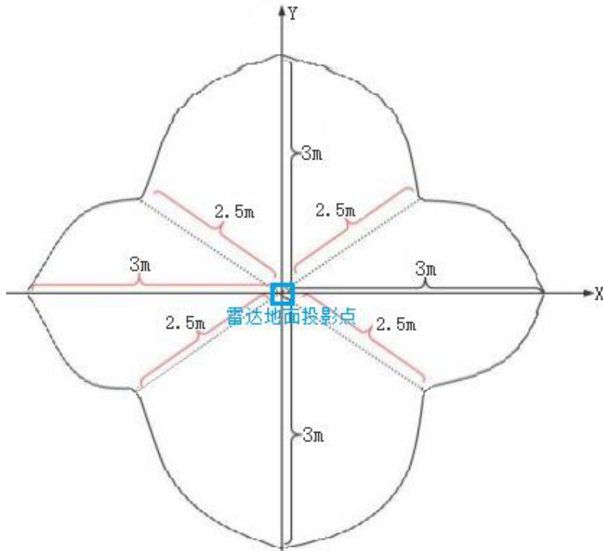
图 3-8 置顶安装极限情况维持范围
