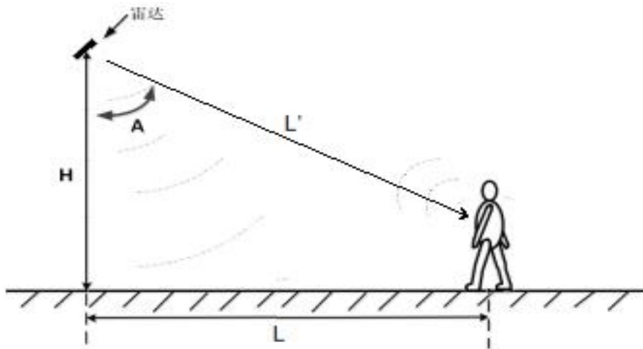
图 3-4 倾斜安装示意图
