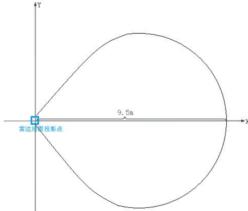
图 3-7 水平安装触发范围
