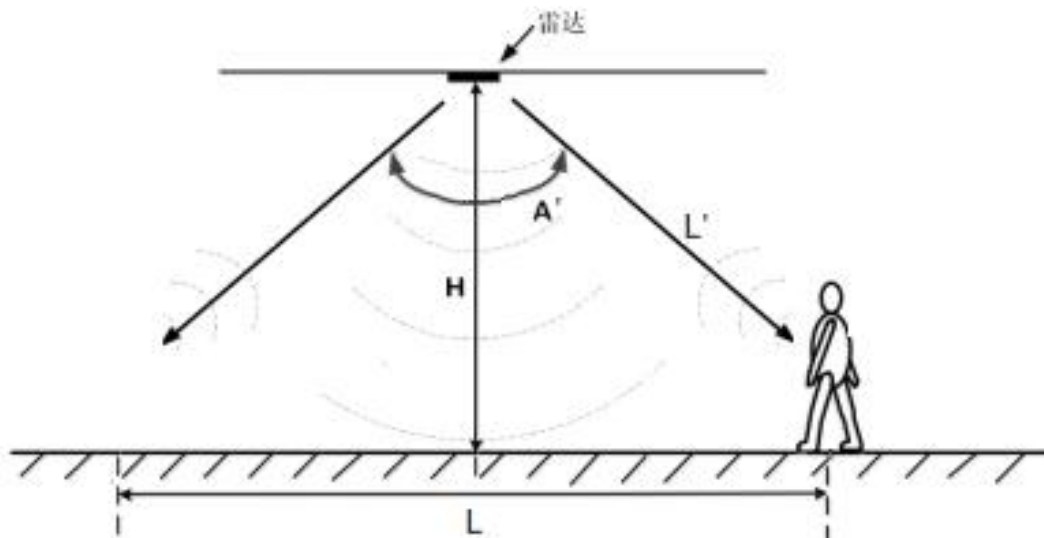
图 3-2 置顶安装示意图
