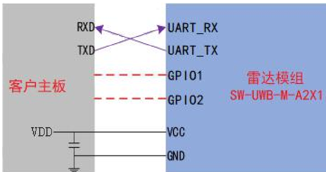
图 2-5 雷达模组连线示意图
