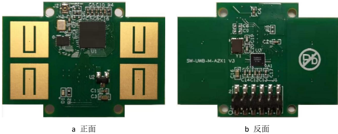
图 2-1 雷达模组实物图
