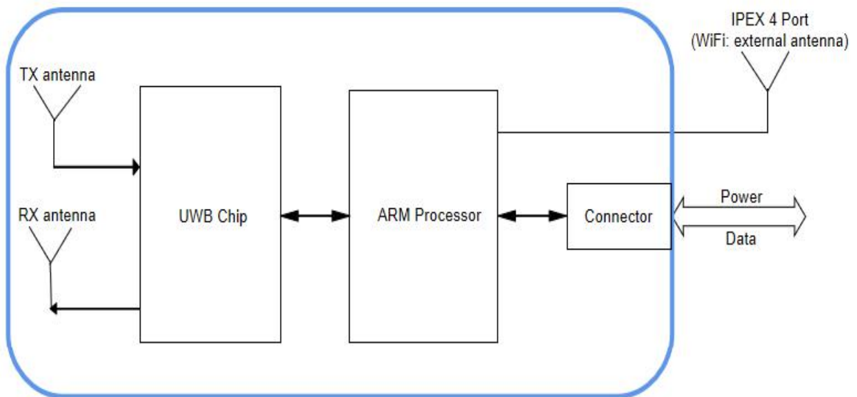
图 1-1 雷达模组方框图
