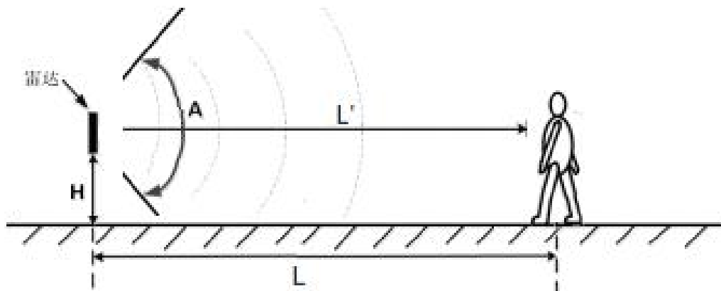
图 3-6 水平安装示意图
