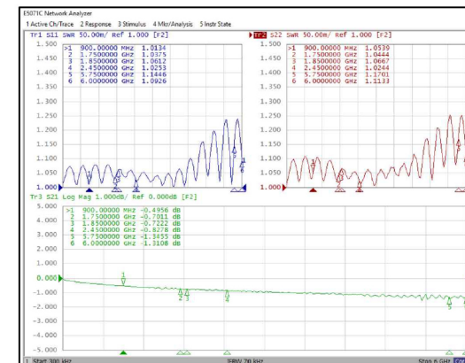
[测试数据: 含350长度线缆]
