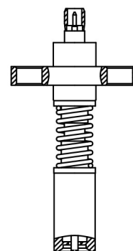
[匹配连接器外形及尺寸]
