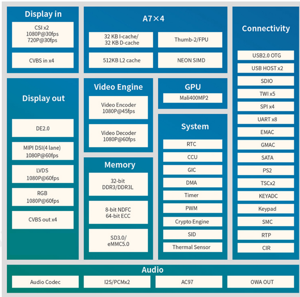
图 6 A40i 处理器功能框图
