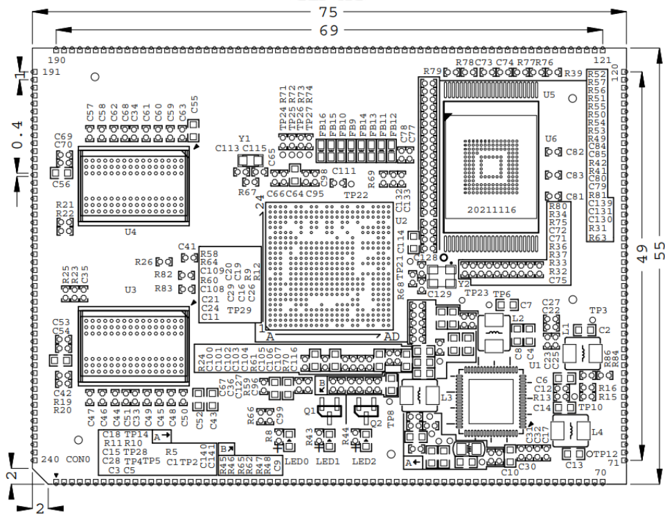
图 7 核心板机械尺寸图
