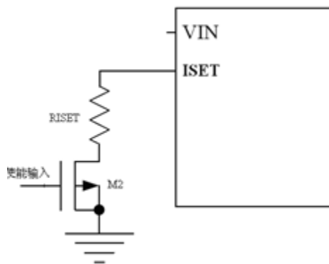
图 5. PL4056 的使能设计
