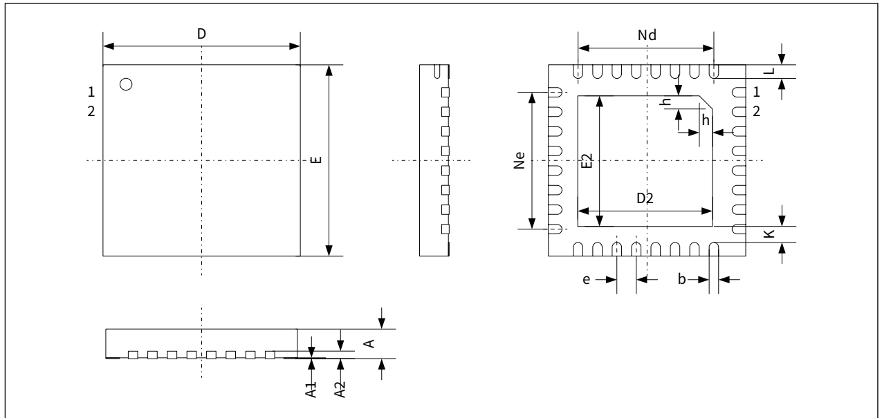
图 8-3 QFN32 引线
