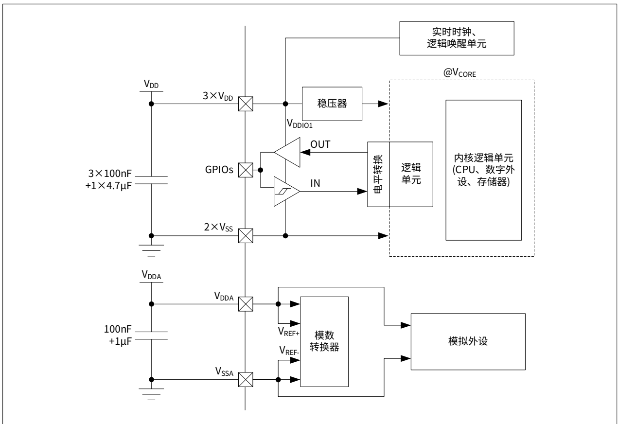
图 7-3 电源系统
