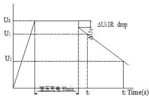
图 2. 充放电曲线图
