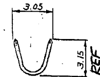
断面 D-D (SECT.)
